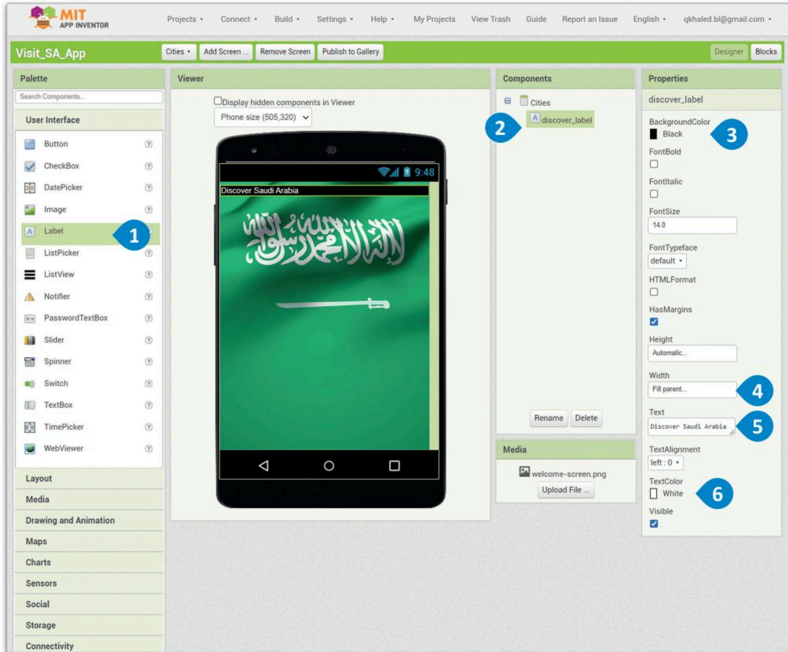
شكل 3.20: إضافة مُكوّن Label ( التسمية )
