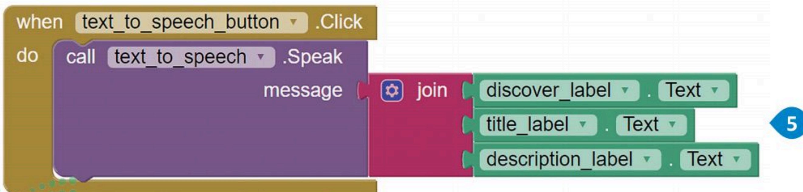
شكل 4.12: برمجة وظيفة تحويل النص إلى كلام
