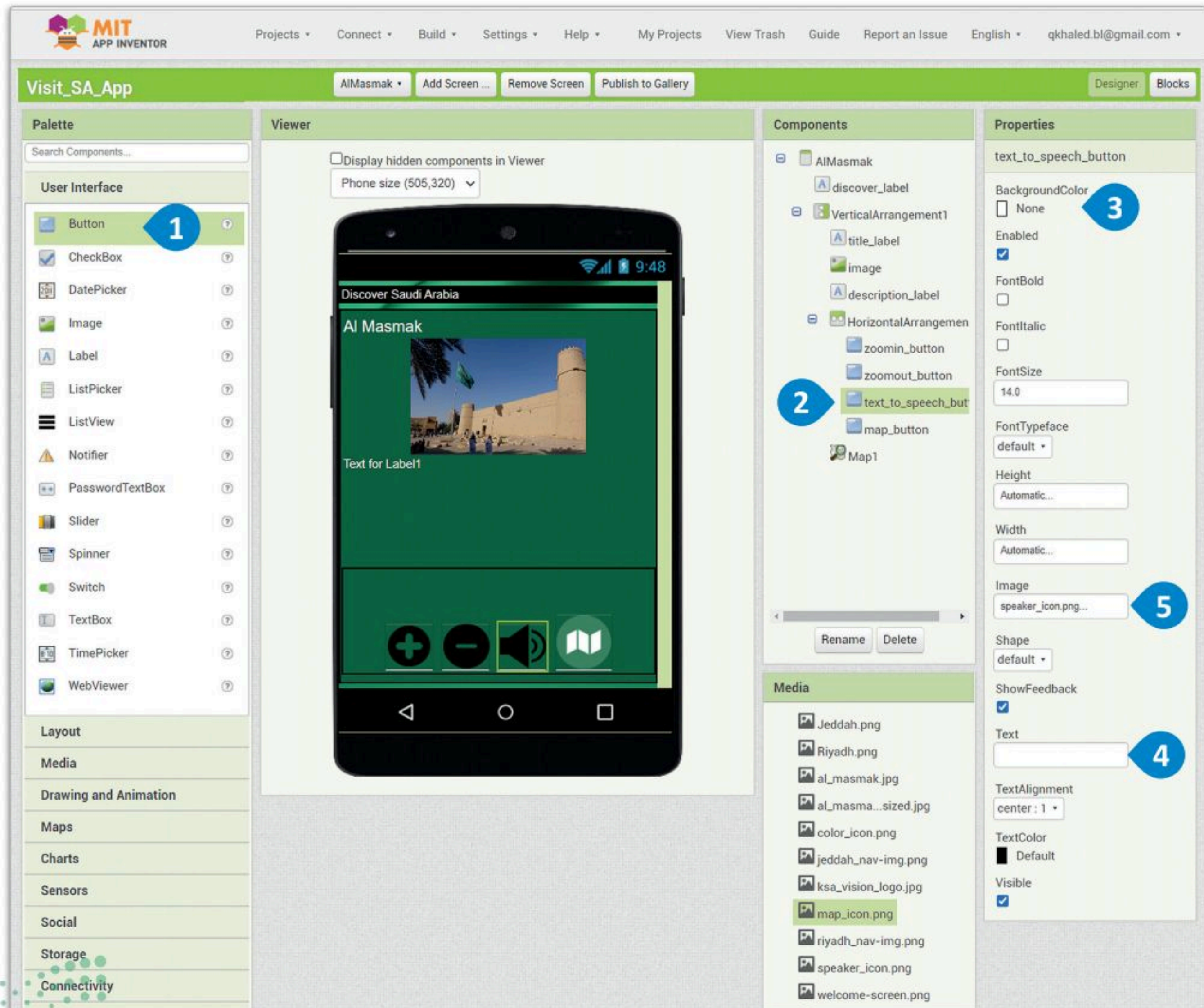
شكل 4.10: إضافة زر تحويل النص إلى كلام
