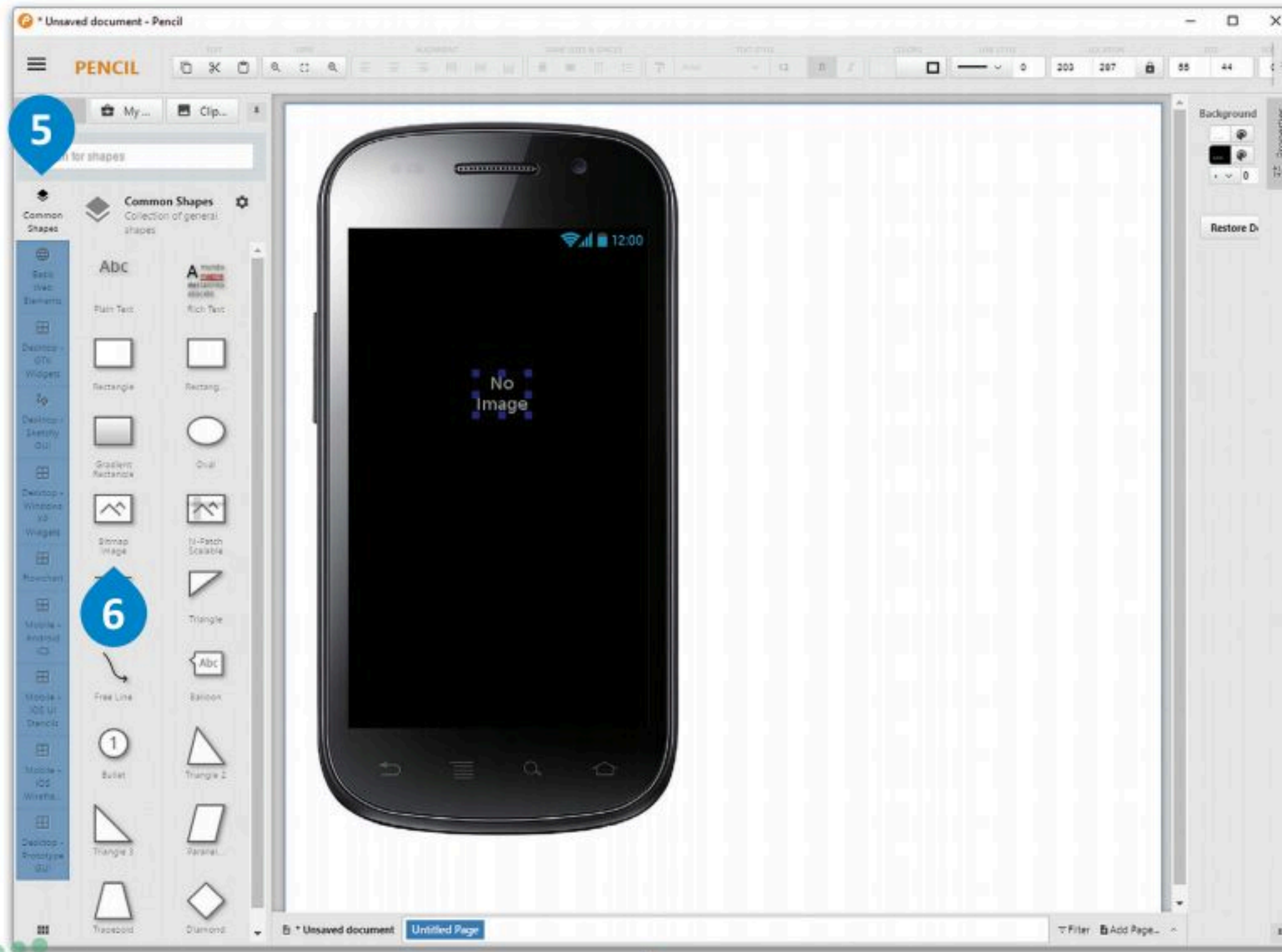
شكل 2.23: إنشاء نموذج أولي جديد باستخدام بنسل
