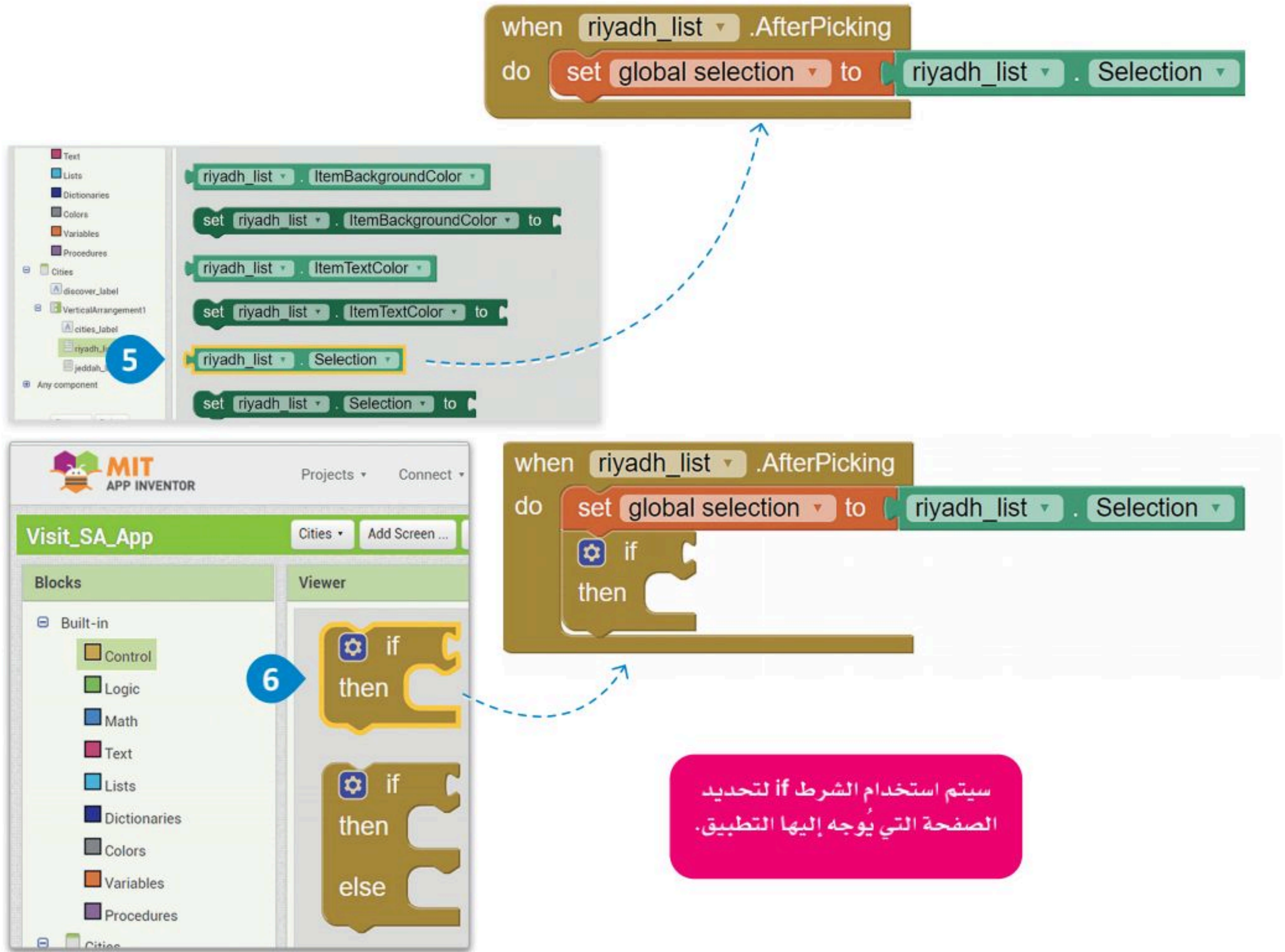
شكل 3.39: تحديد الصفحة من ListPicker (قائمة الخيارات)
