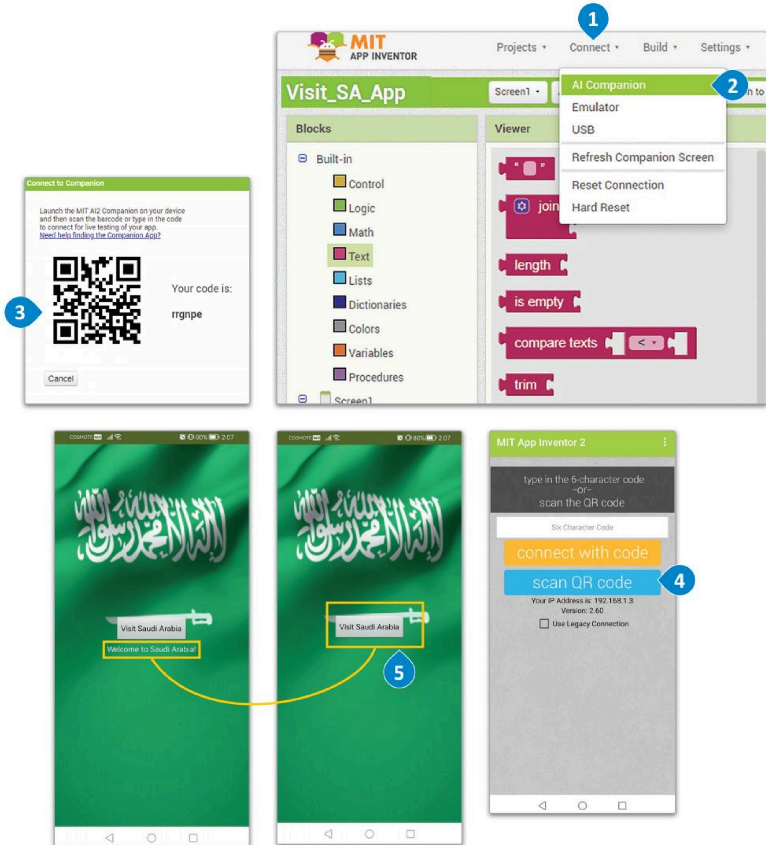
شكل 3.16: اختبار التطبيق باستخدام MIT AI2 Companion
