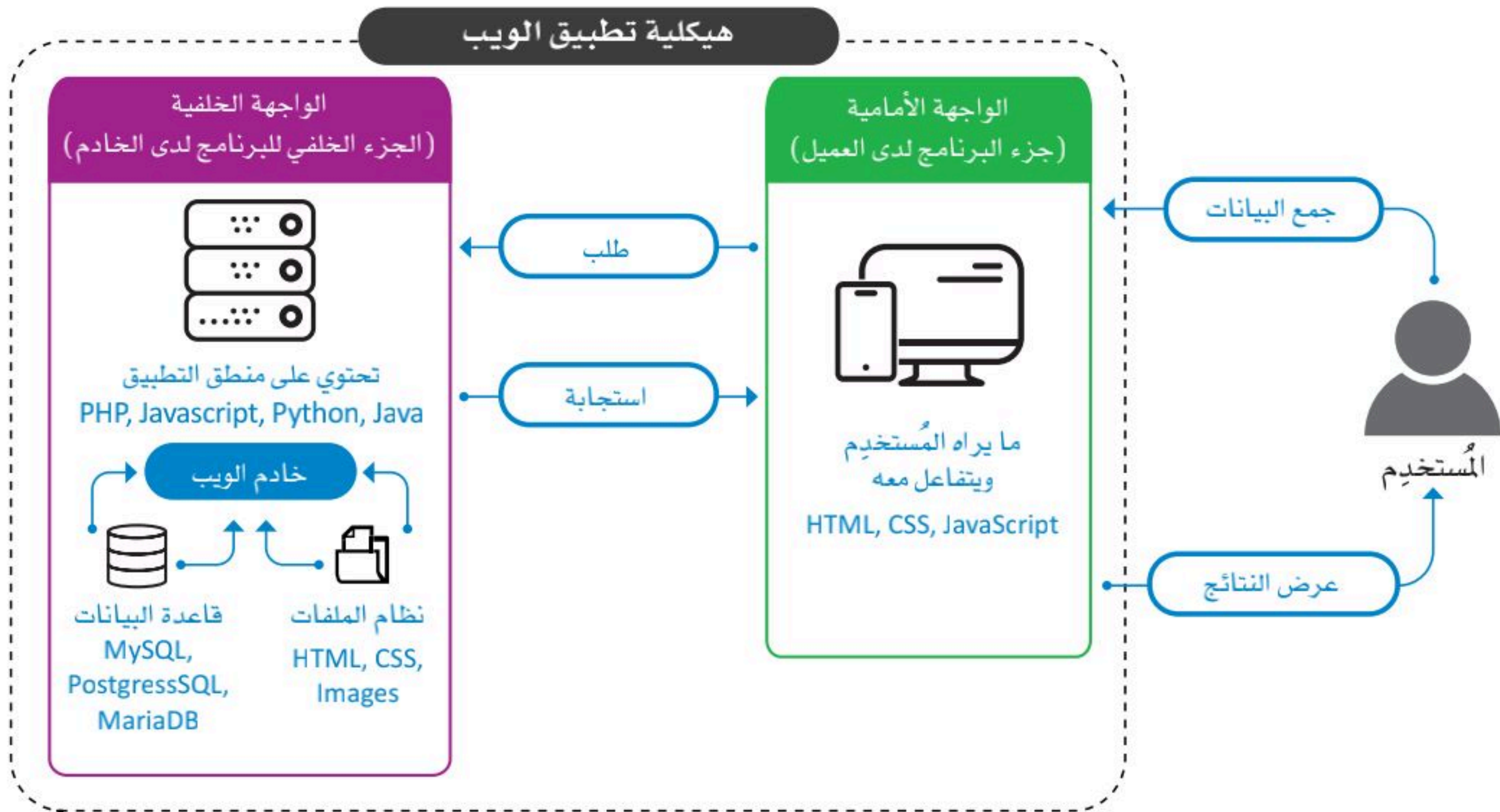
شكل 1.20: الهيكلية الأساسية لتطبيق الويب
