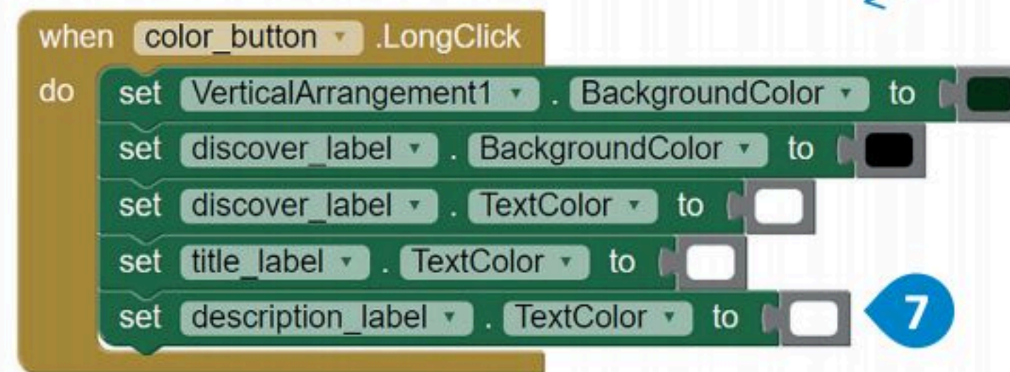
شكل 4.14: برمجة زر نسق اللون
