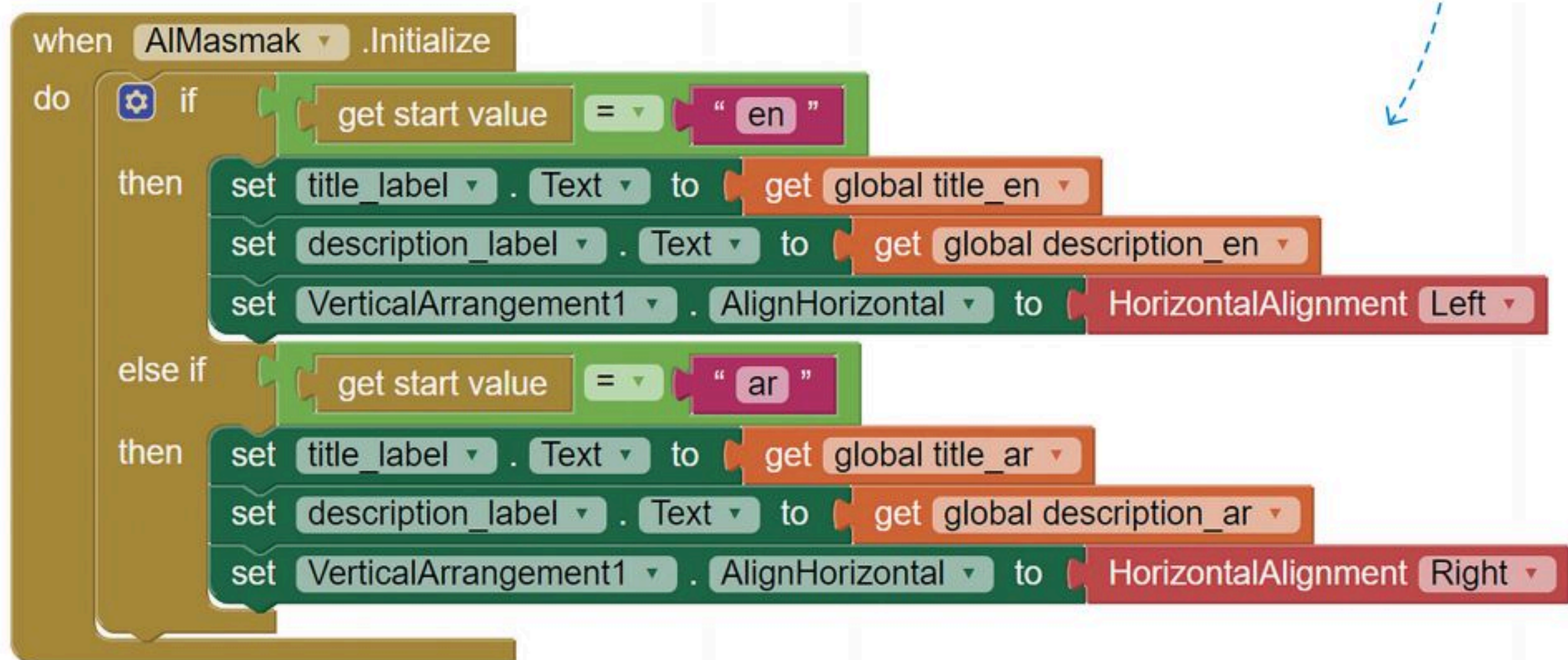
شكل 3.42: تغيير اللغة ديناميكياً
