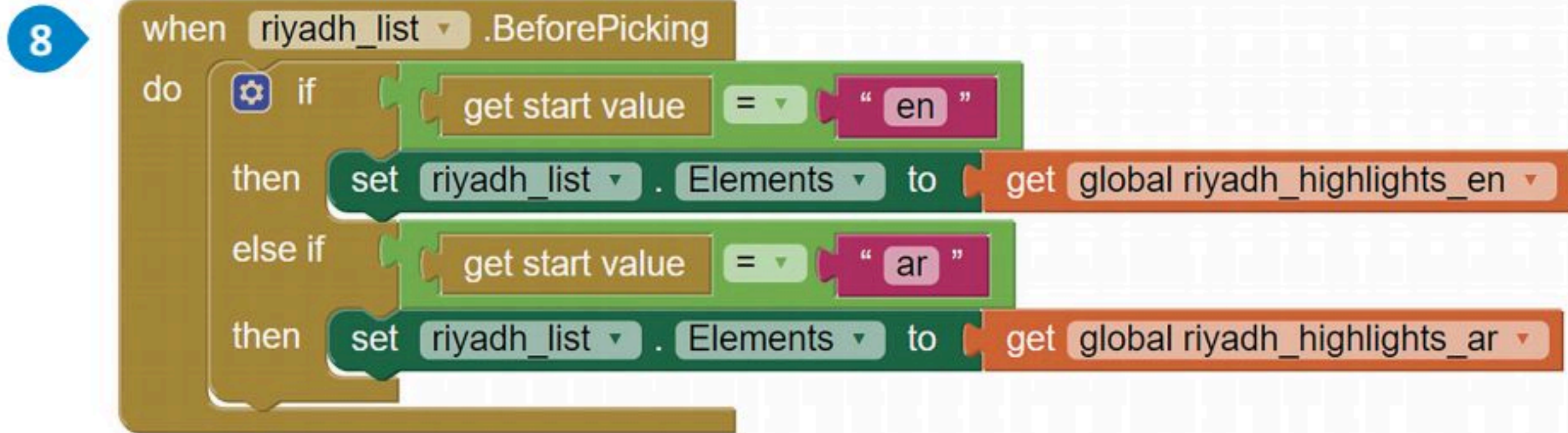
شكل 3.38: تهيئة محتوى ListPicker (قائمة الخيارات)
