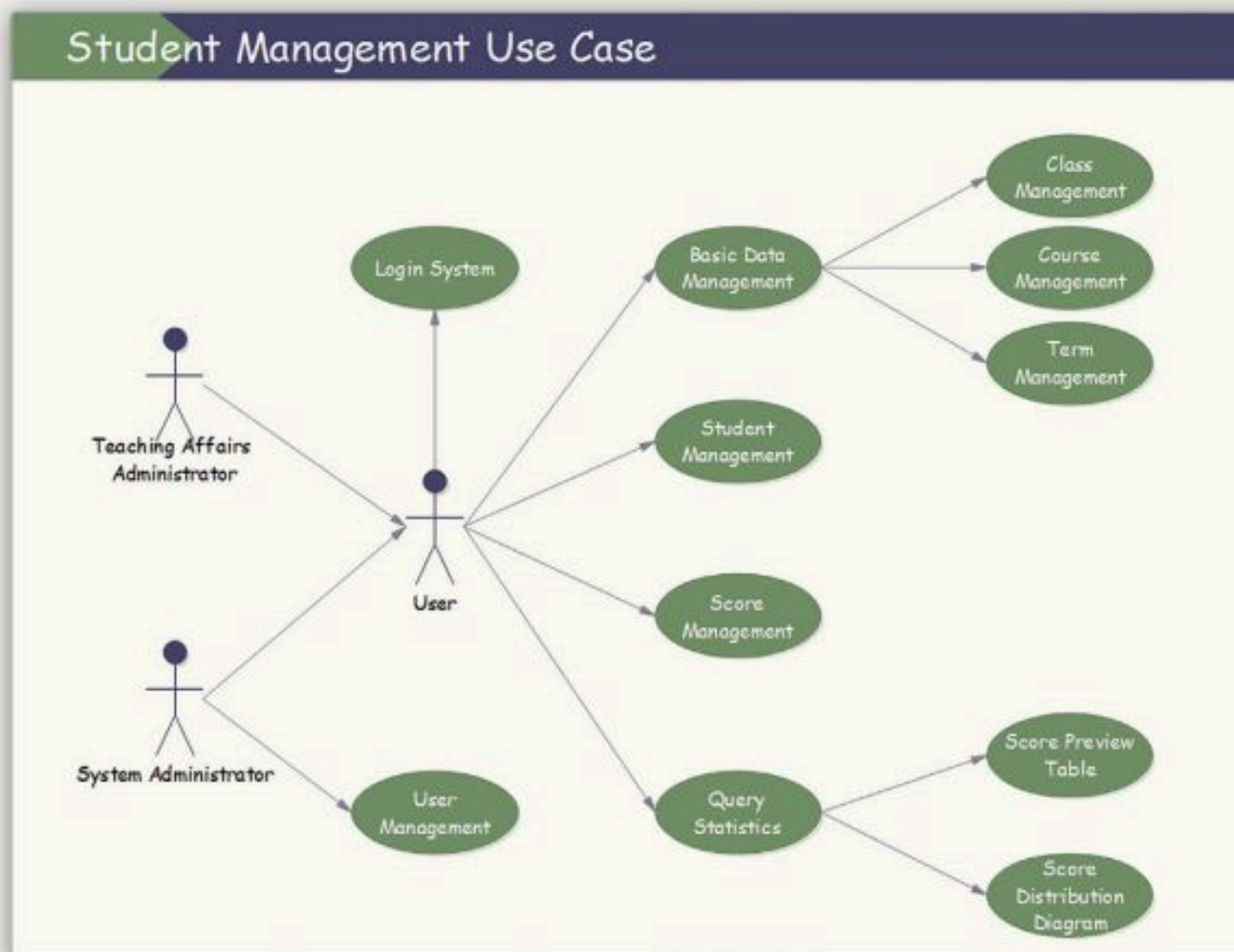
شكل 2.5: مخطط حالة الاستخدام
