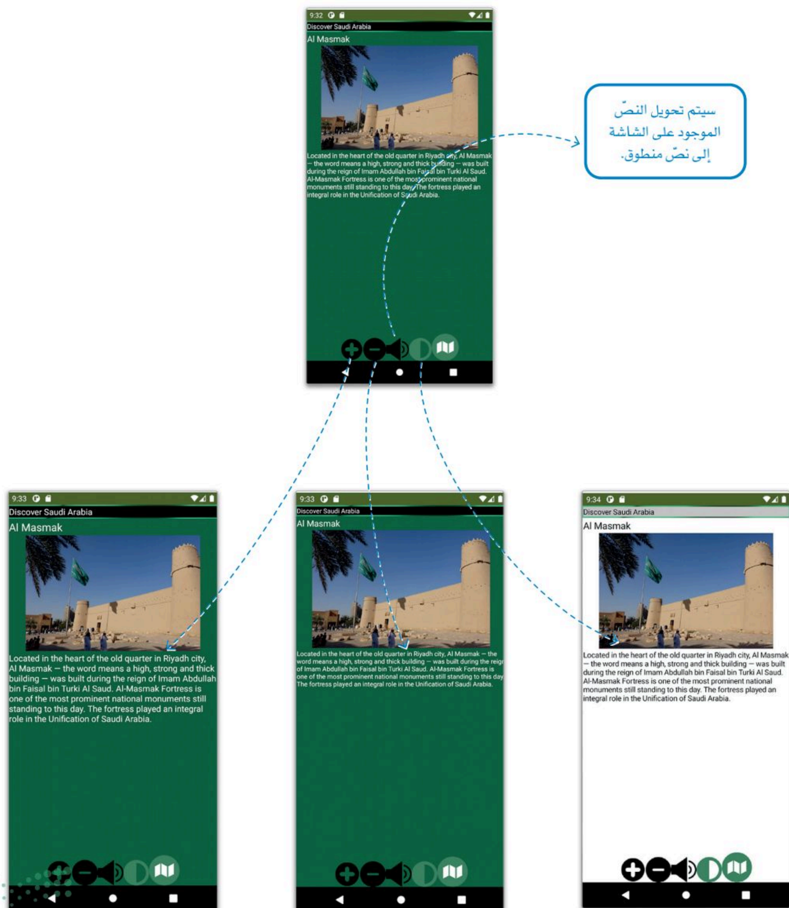
شكل 4.15: ميزات قابلية الوصول في المحاكي
