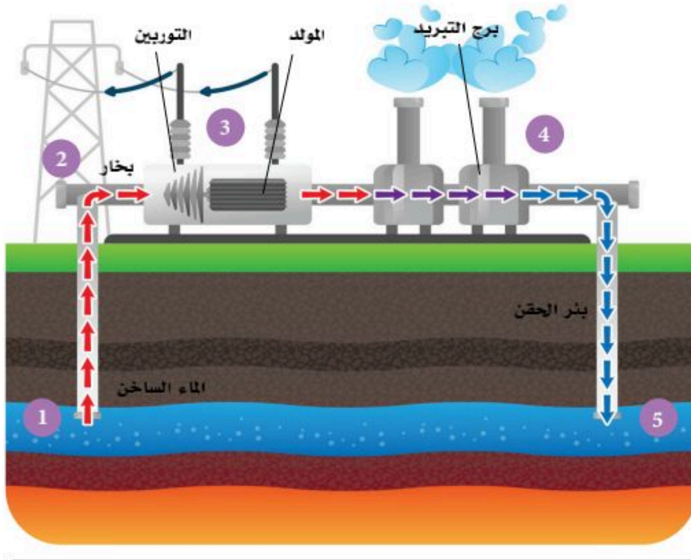
الشكل 10-5 الطاقة الحرارية الأرضية.
