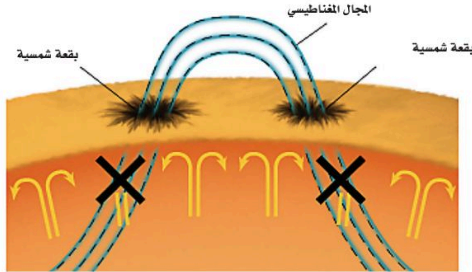
الشكل 2-7 التواء خطوط المجال المغناطيسي بسبب الدوران التفاضلي للشمس ونشوء البقع الشمسية.
