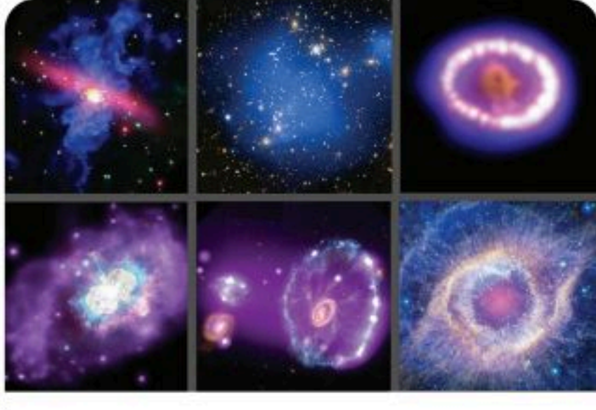
الشكل 17-3 صور لـ سد م نطاق الأشعة السينية بواسطة مرصد شاندرا. المصدر: وكالة ناسا.
