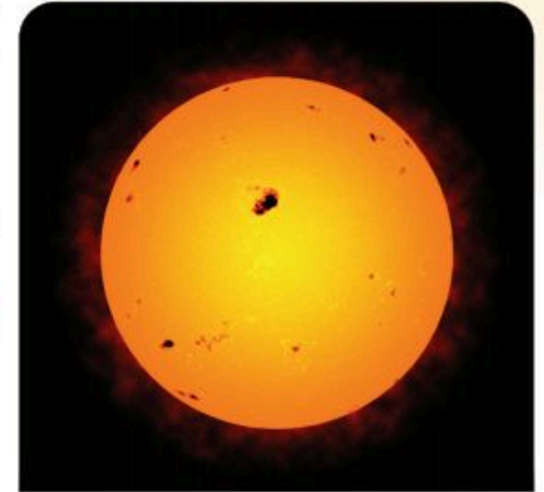
الشكل 2-8 البقع الشمسية على سطح الشمس.
