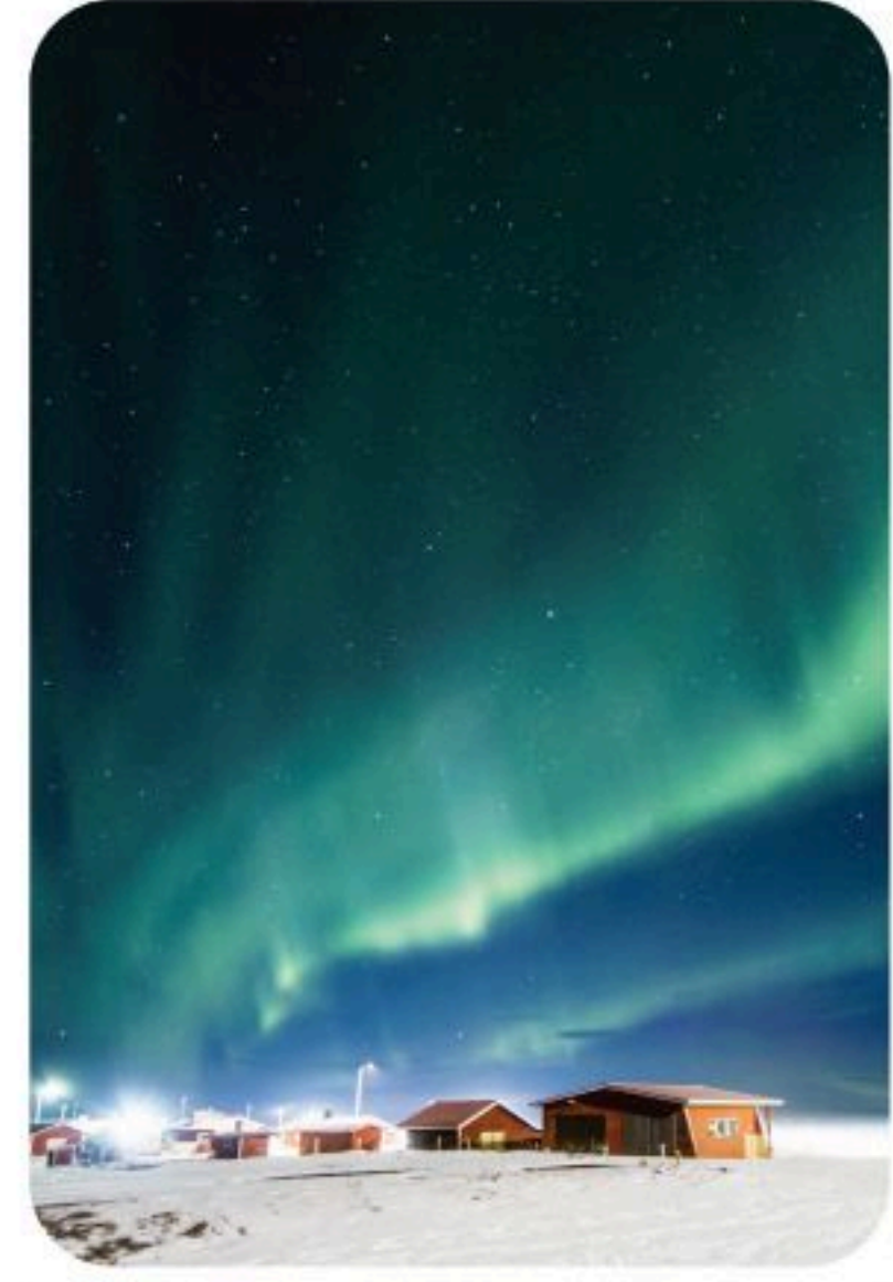
الشكل 12-2 الشفق القطبي.
