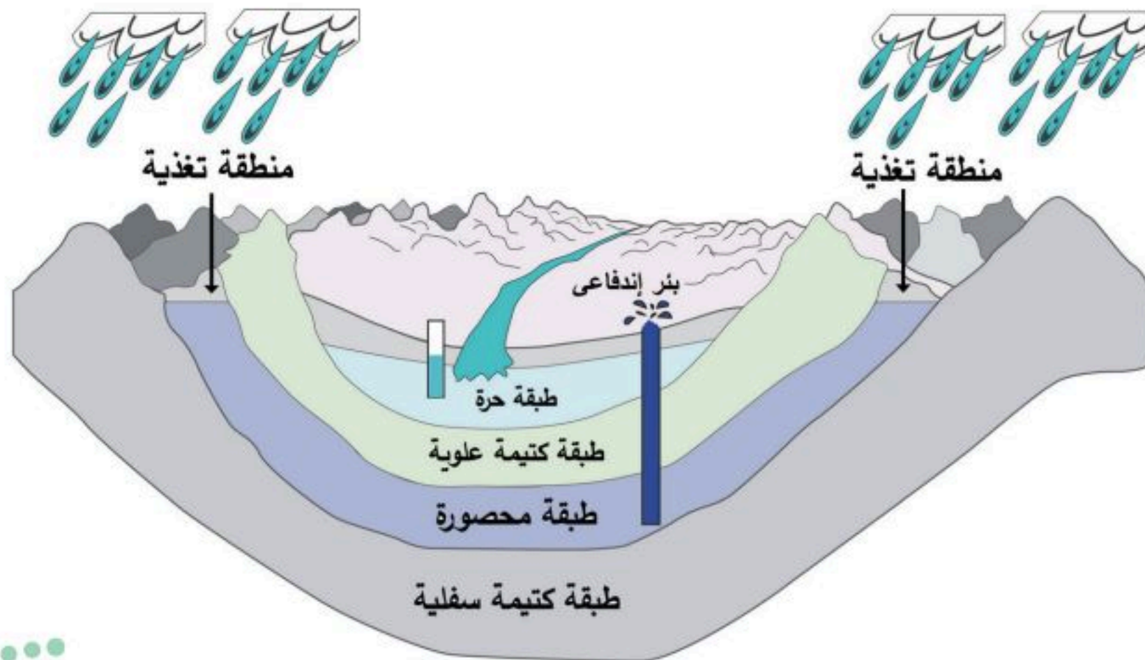
الشكل 16-6 الطبقة المحصورة.
