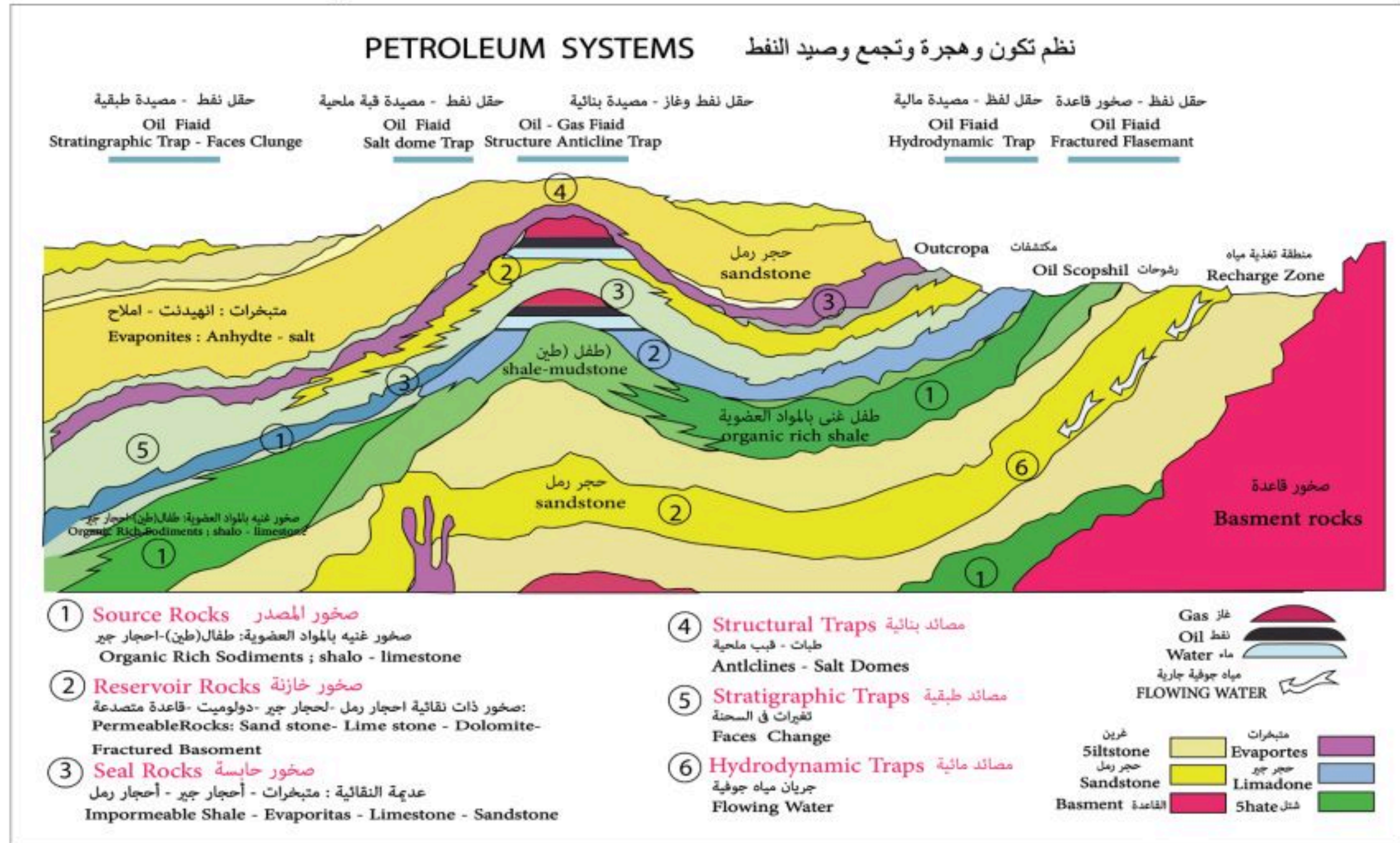
الشكل 1-5 النظام النفطي.
