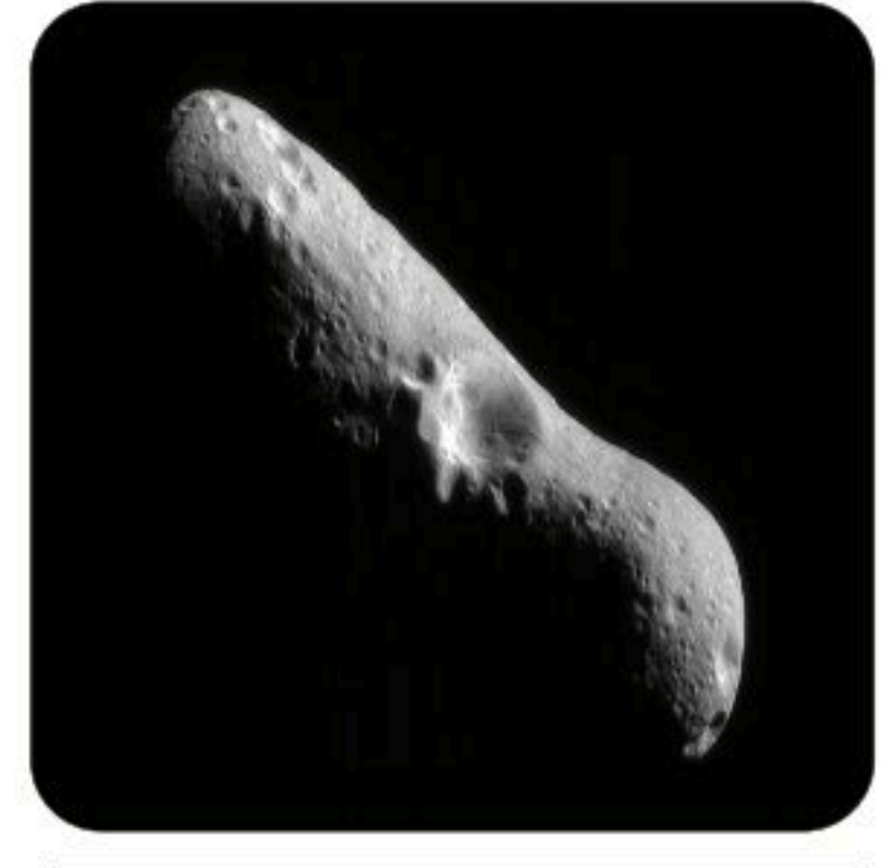
الشكل 12-1 صورة لكويكب إيروس.
