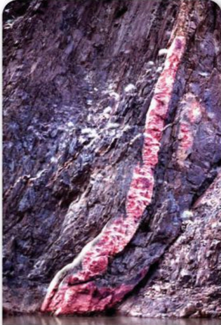
الشكل 20-4 بحسب مبدأ القاطع والمقاطع فإن القواطع النارية أحدث من صخور الشيست.
