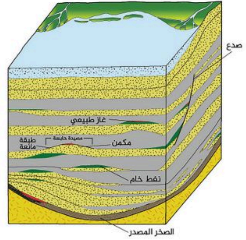
الشكل 2-5 صخر المصدر.
