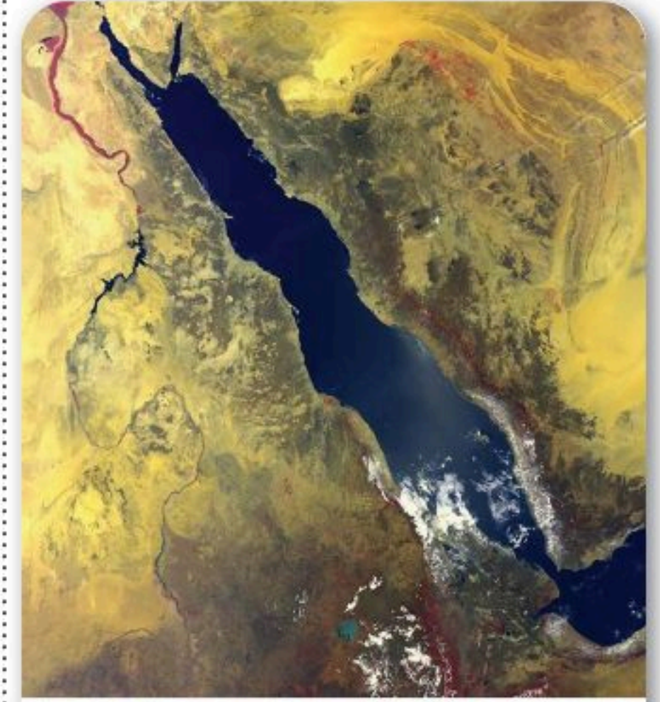
الشكل 6-7 البحر الأحمر ويتضح على جانبية الدرّ العربي والدرّ النوبي.
