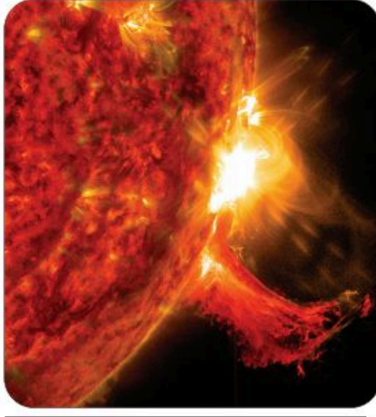
الشكل 9-2 التوهجات الشمسية.
