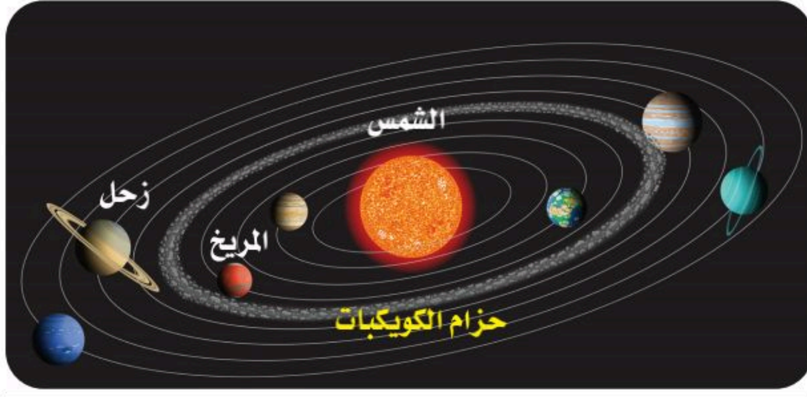
الشكل 11-1 موقع حزام الكويكبات.
