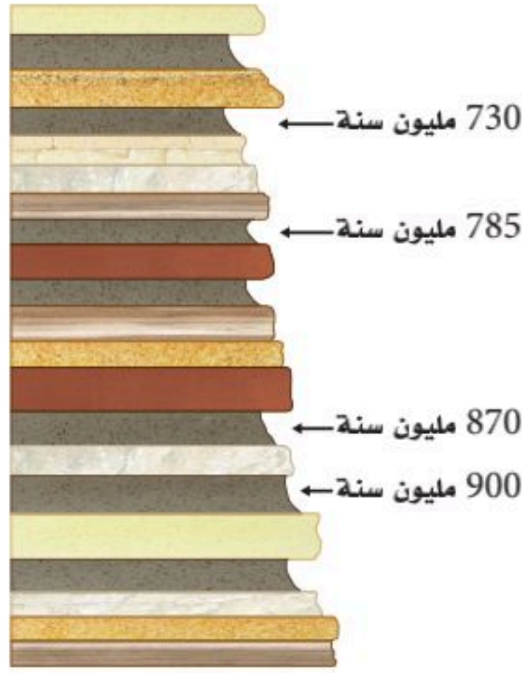
تأريخ الرماد البركاني إشعاعياً
