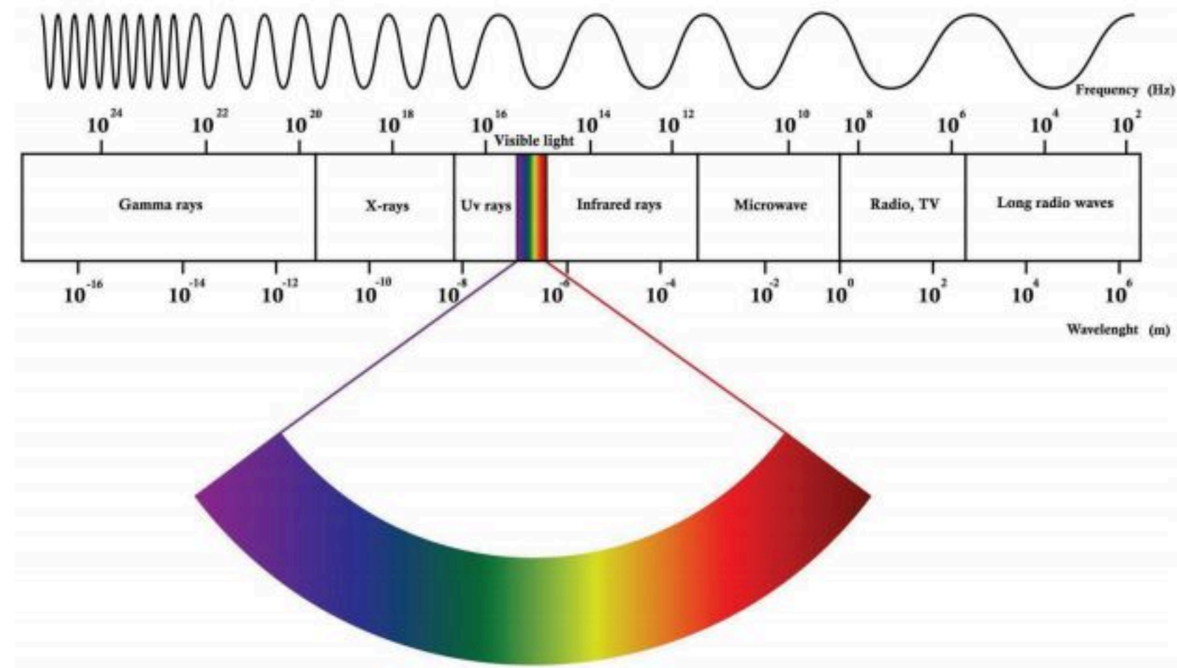
الشكل 1-3 نطاقات الطيف الكهرمغناطيسي.
