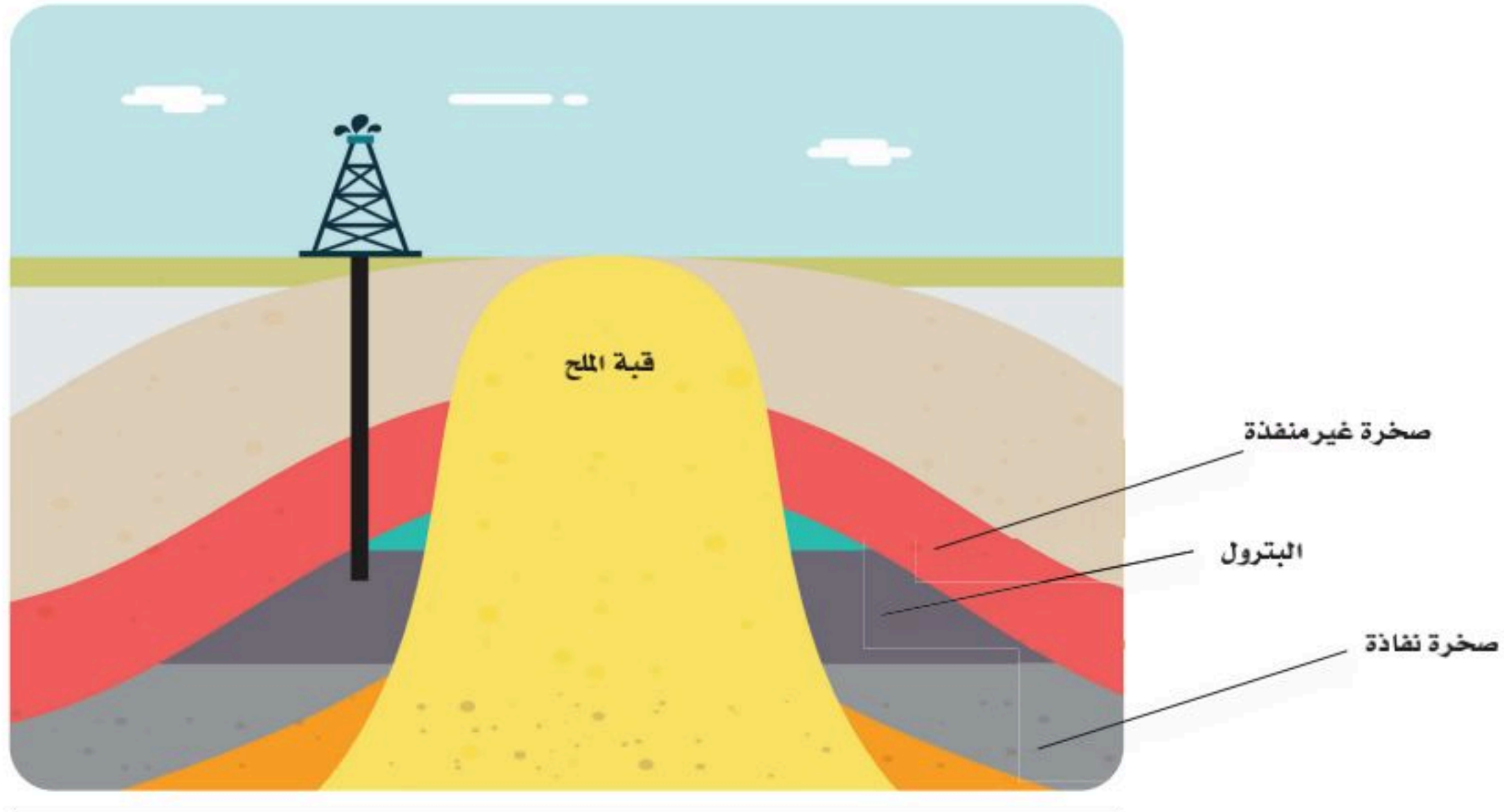
الشكل 5-5 مصائد القباب الملحية.
