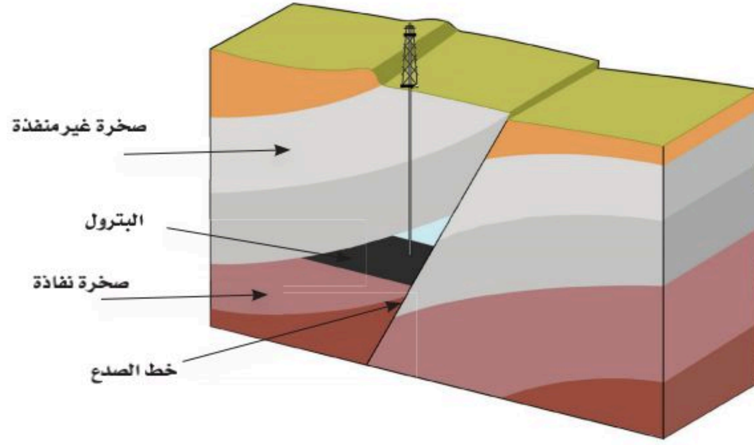
الشكل 4-5 مصائد الصدوع.
