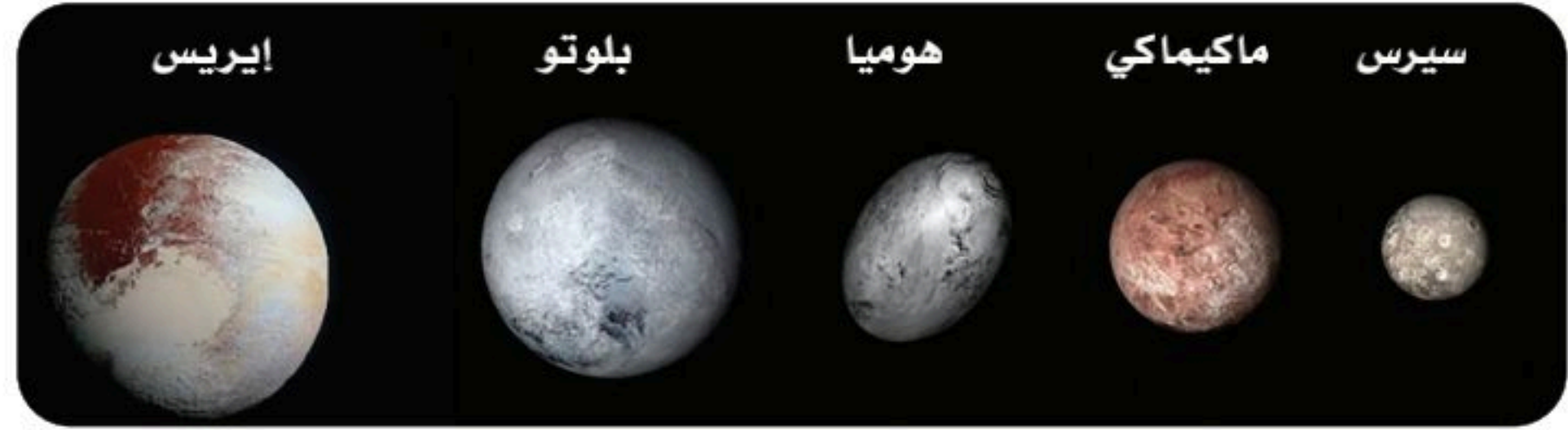
الشكل 2-1 الكواكب القزمة في نظامنا الشمسي.
