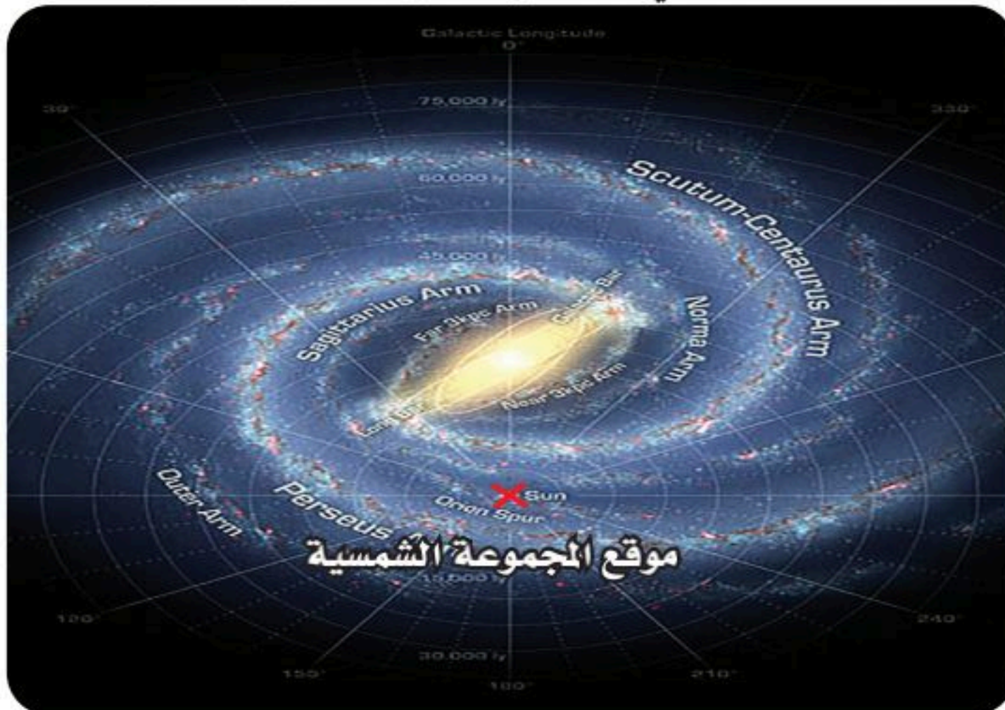
الشكل 1-1 صورة افتراضية لموقع المجموعة الشمسية في أحد أذرع مجرة درب التبانة.
