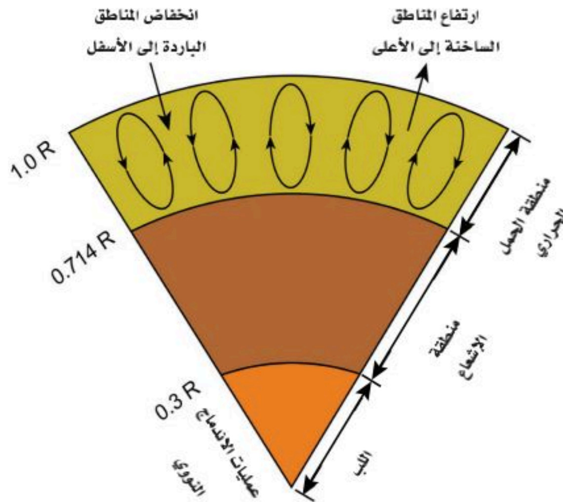
الشكل 2-3 التركيب الداخلي للشمس.
