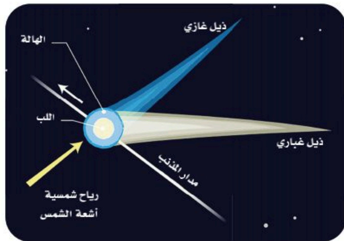
الشكل 20-1 تركيب المذنبات.
