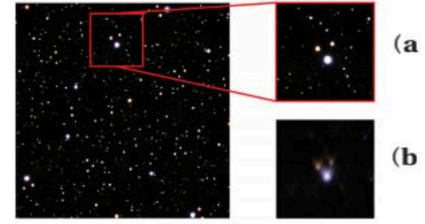
الشكل 10-3 صورة توضح الزيف الهالي.
