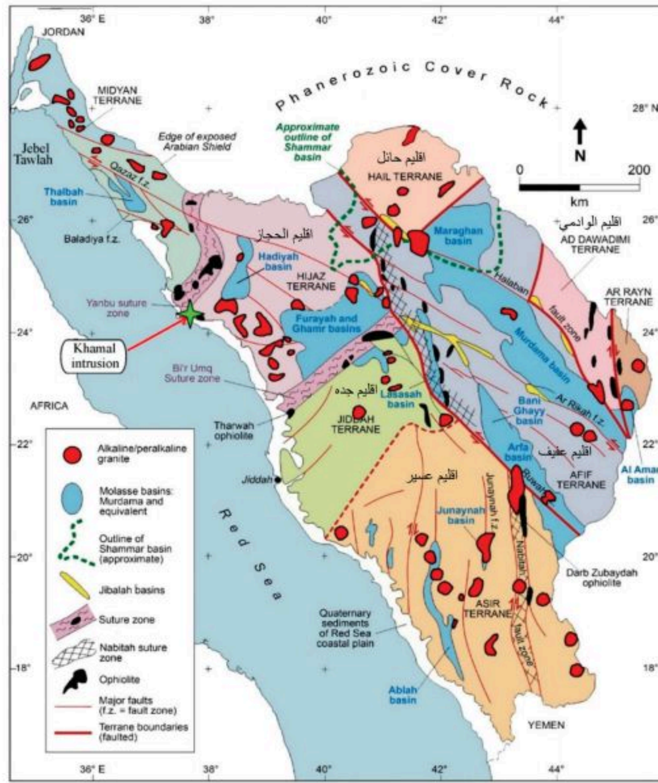
الشكل 3-6 خريطة توضح مواقع أقاليم الدرع العربي.
