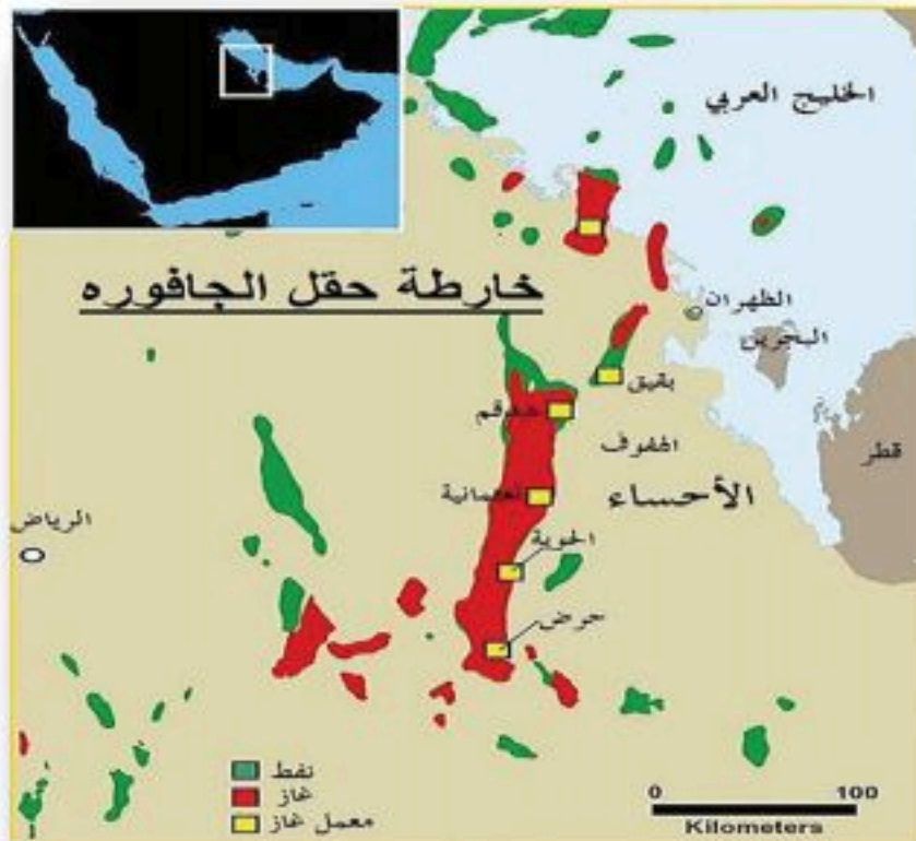
خارطة حقل الجافورة الجيولوجية.
