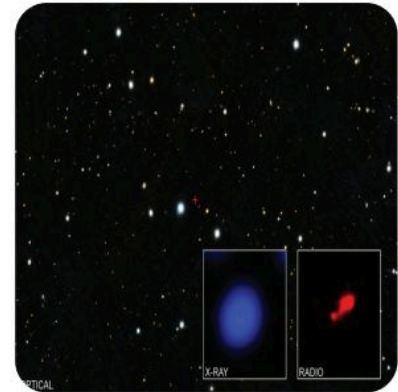
الشكل 16-3 كوازارات.
