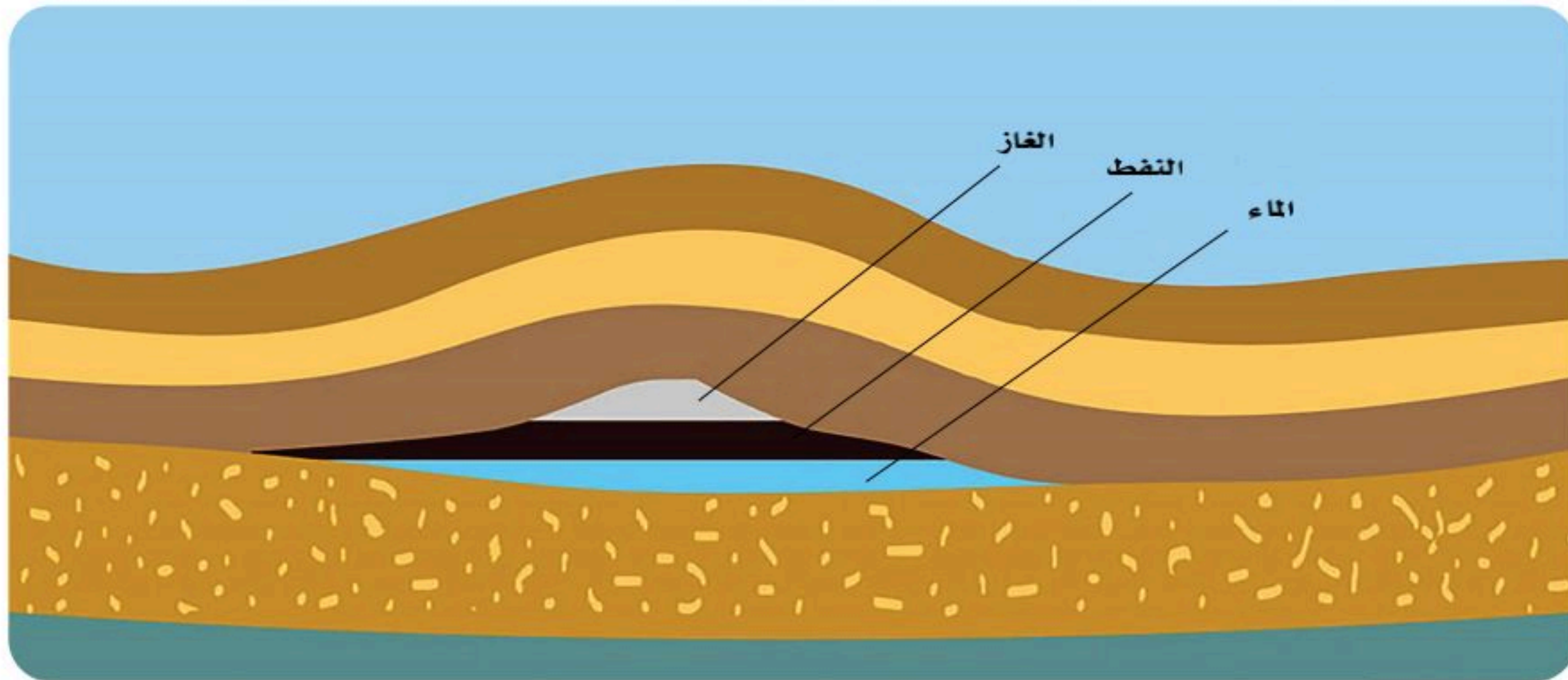
الشكل 3-5 مصائد الطيات المحدبة.
