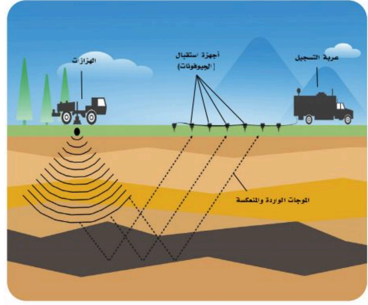
الشكل 5-7 المسح الزلزالي.
