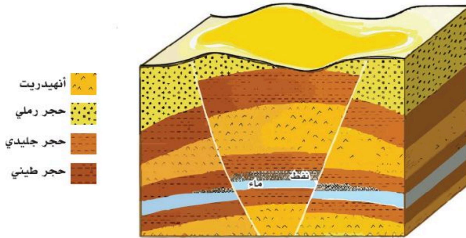
الشكل 6-5 المصائد المركبة.
