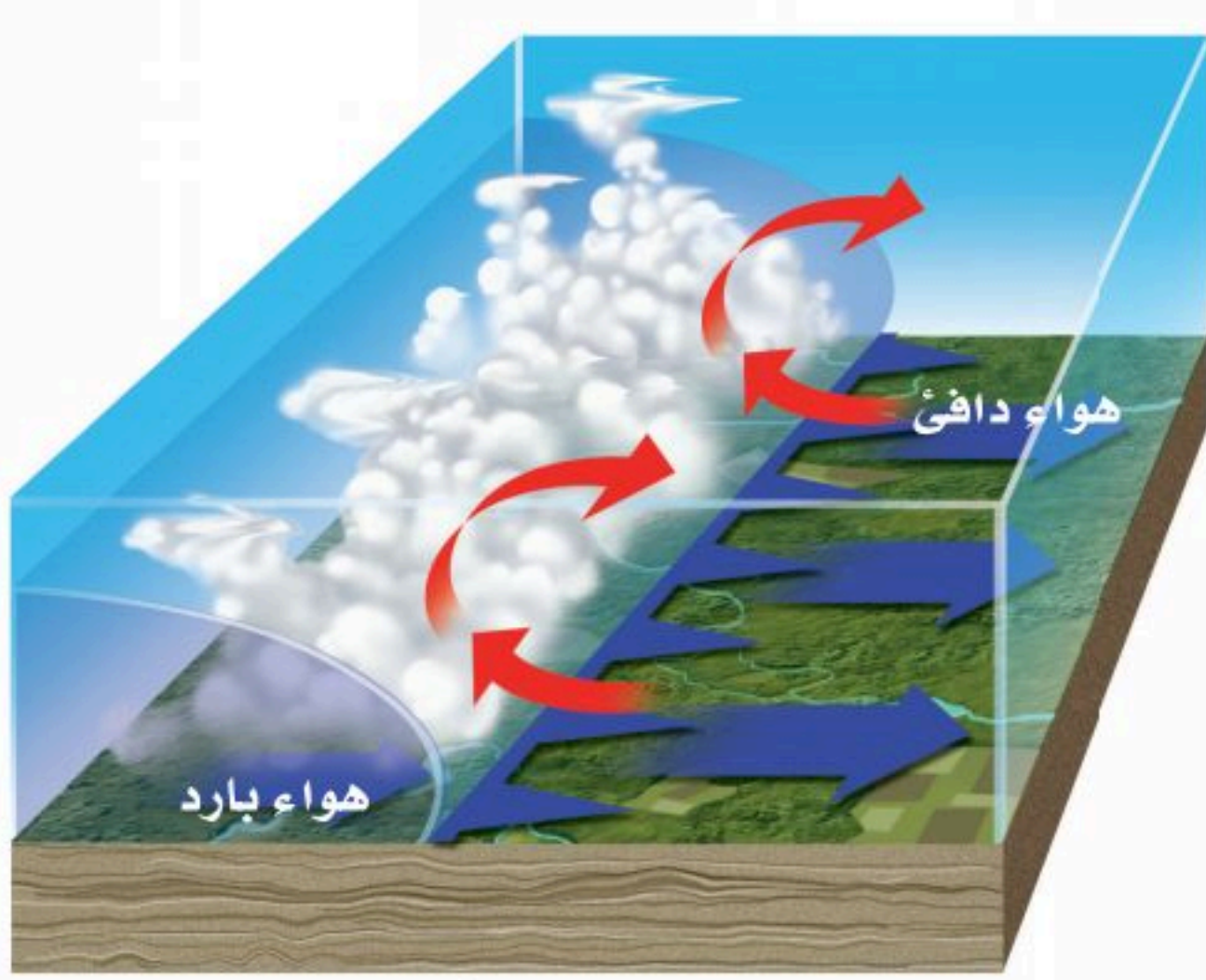
تشكل جبهة باردة
