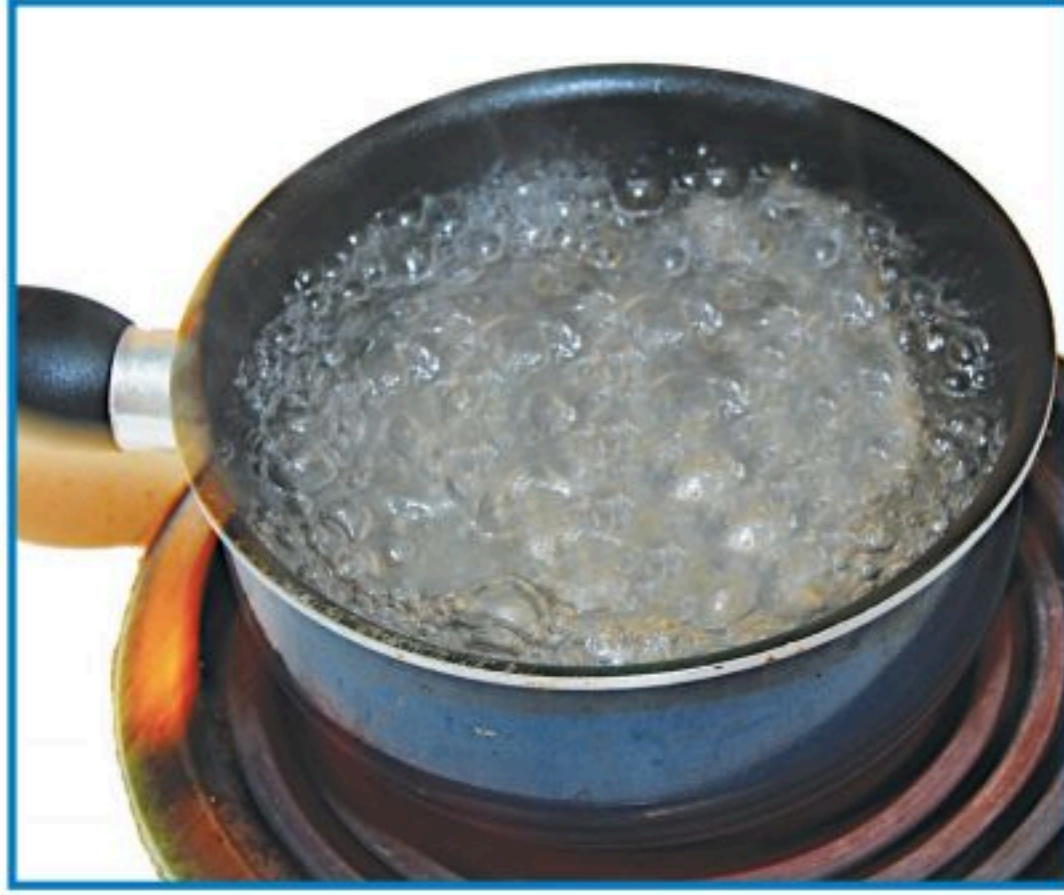
يزداد التبخر عند درجة الغليان
