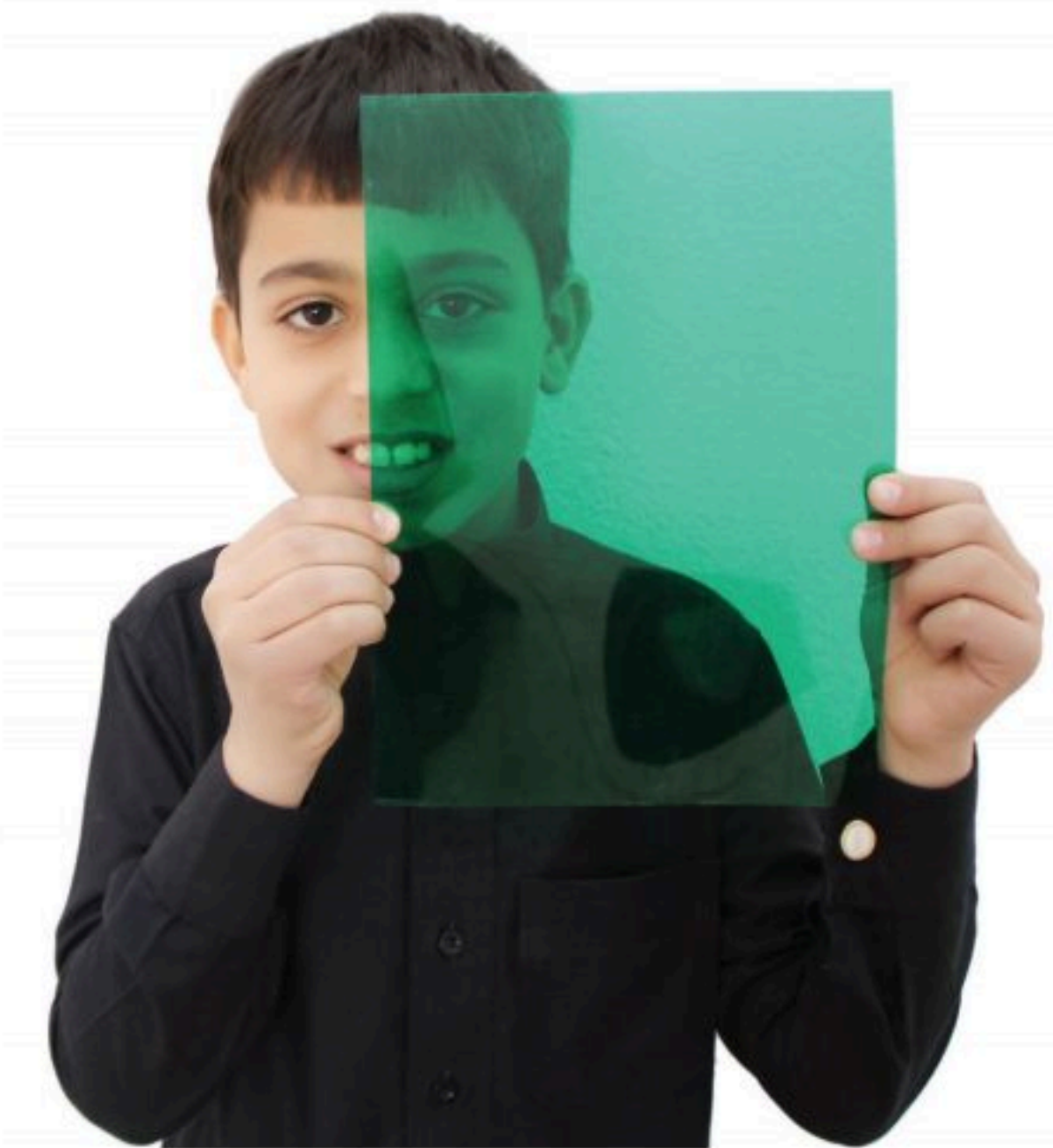
الجسم شبه الشفاف يمرر جزءًا يسيرًا من الضوء.
