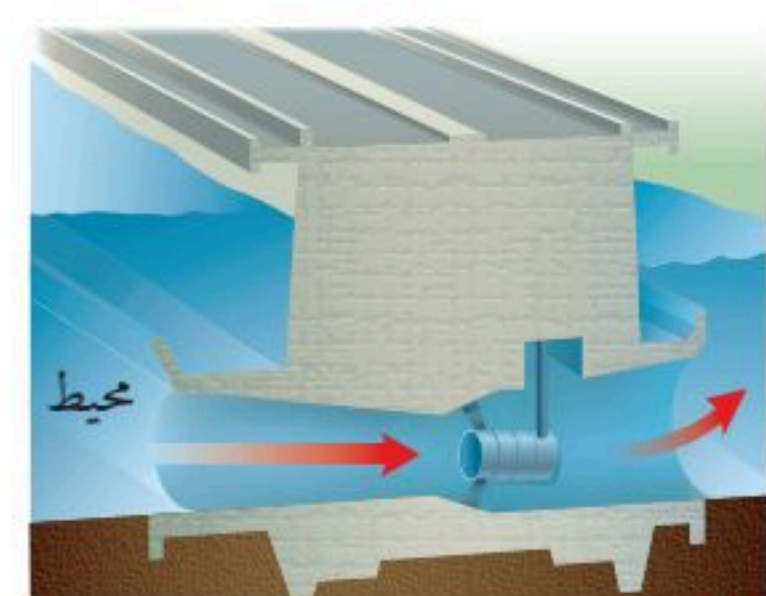
أ خلال المد تدير حركة الماء التوربين المرتبط مع المولد الكهربائي، وعند اكتمال المد تغلق البوابة لتحجز الماء خلف السد.
