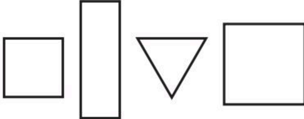
٤ مُرَبَّعٌ
