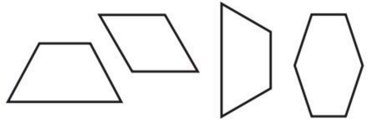
٣ شِبْهُ مُنْحَرَفٍ
