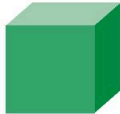
مُكْعَبٌ
