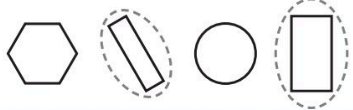
١ مُسْتَطِيلٌ
