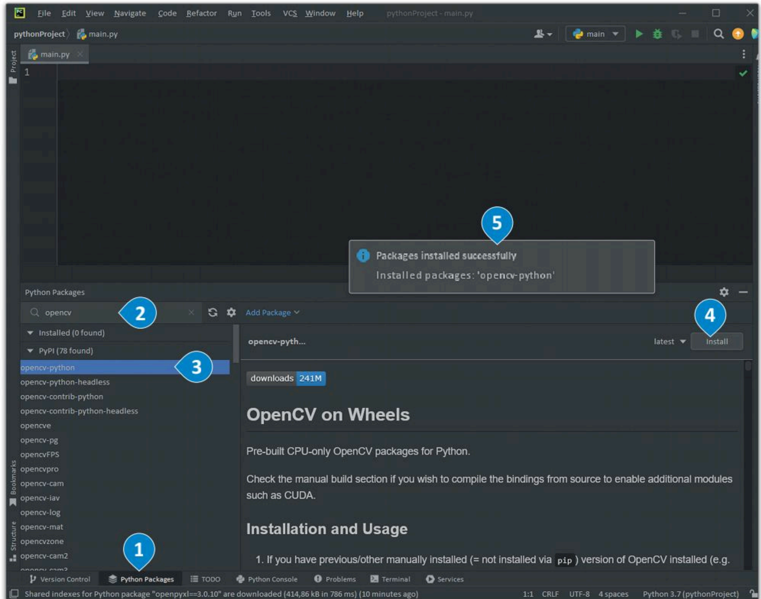
شكل 6.8: تثبيت مكتبة أوبن سي في
