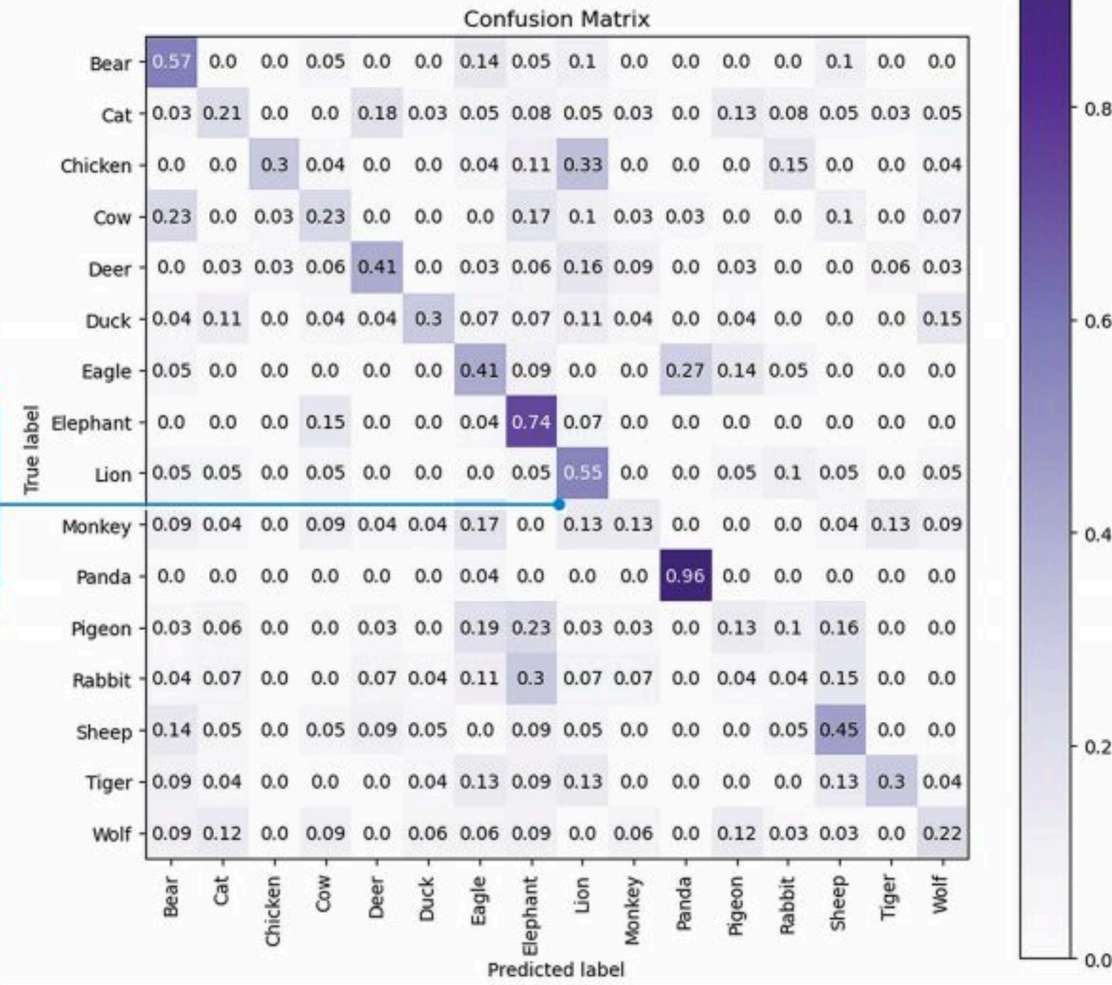
شكل 4.7: مصفوفة الدقة الخاصة بأداء خوارزمية MultinomialNB
