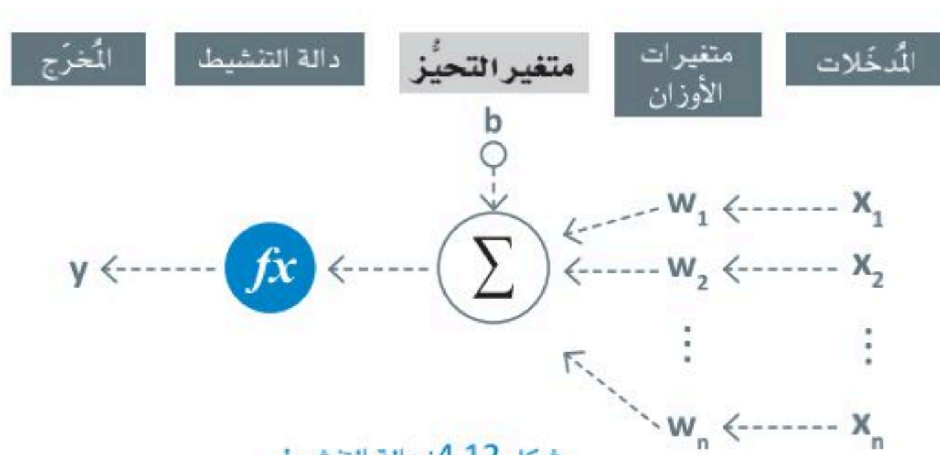
شكل 4.12: دالة التنشيط
