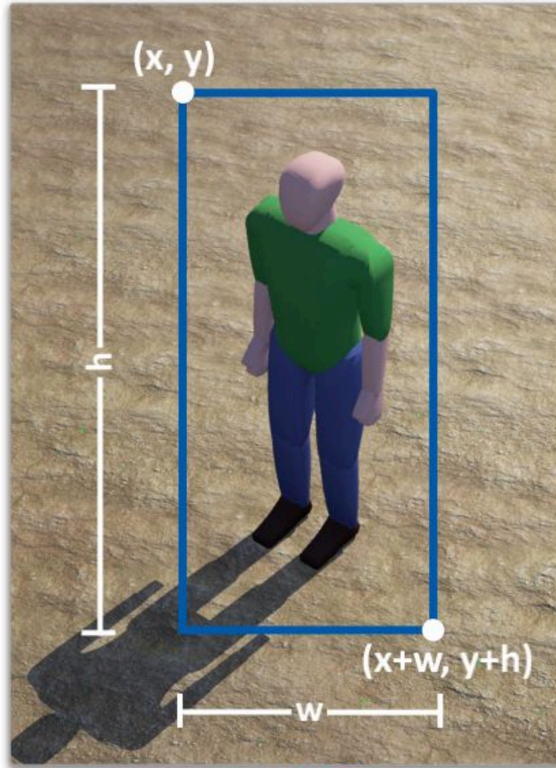
شكل 6.20: متغيرات المستطيل
