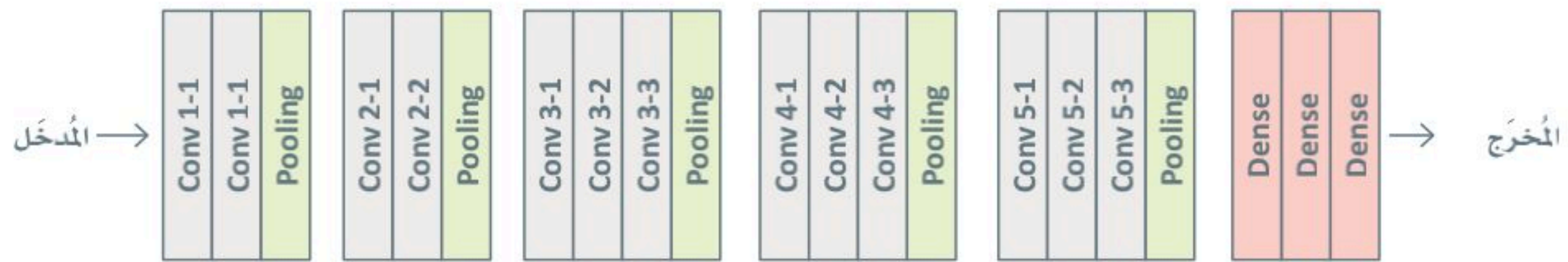
شكل 4.22: معمارية نموذج VGG16
