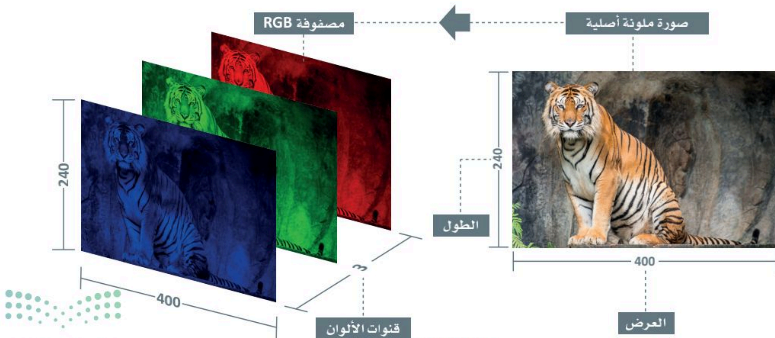
شكل 6.18: أبعاد الصورة
