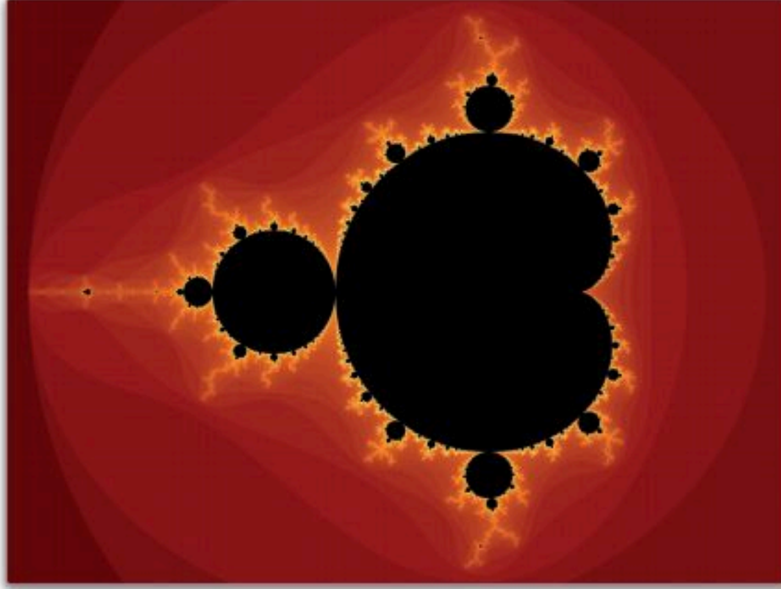
شكل 4.25: فراكتل ماندلبروت
