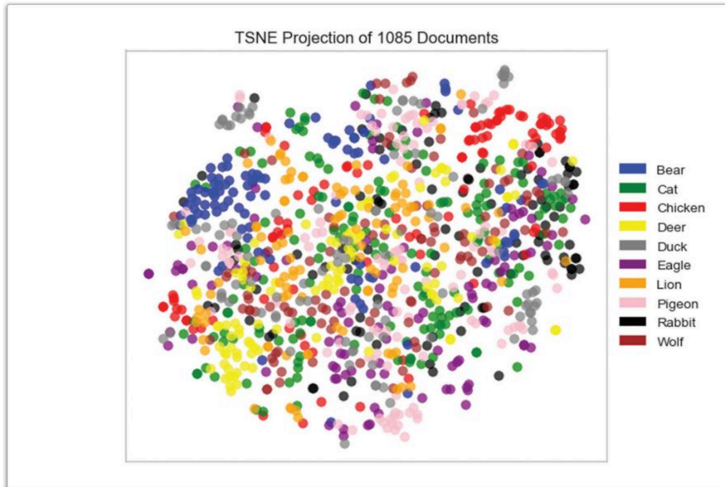
شكل 4.18: تصوير العناقيد
