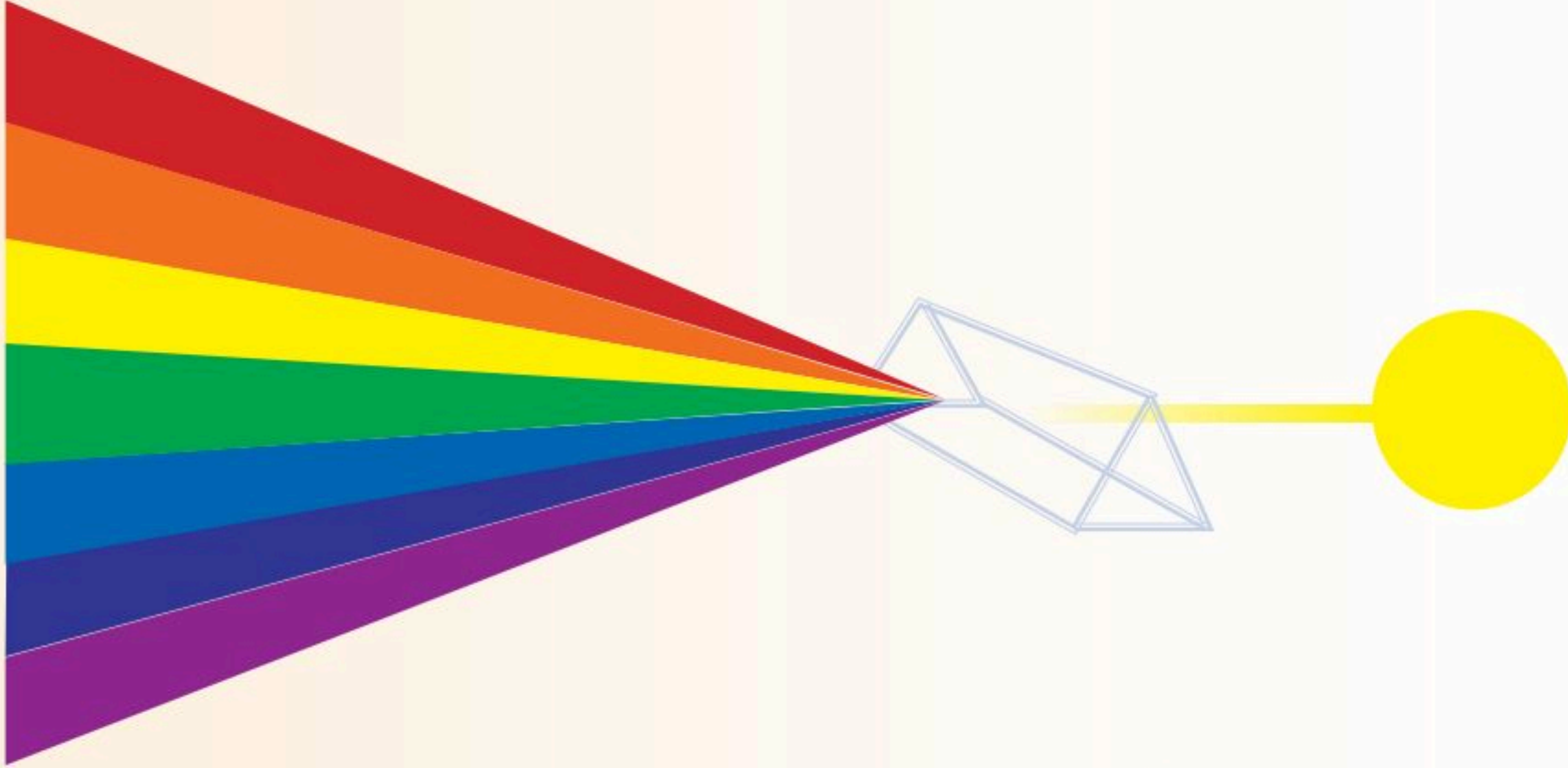
شكل (١): ظاهرة الانكسار وألوان الطيف.
