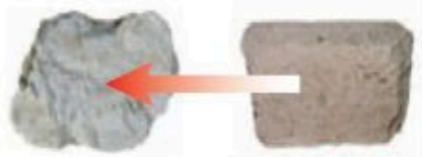
ج الحجر الجيري يتحول إلى رخام.
