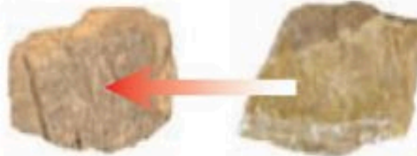
ب الرمل يتحول إلى كوارتزيت.
