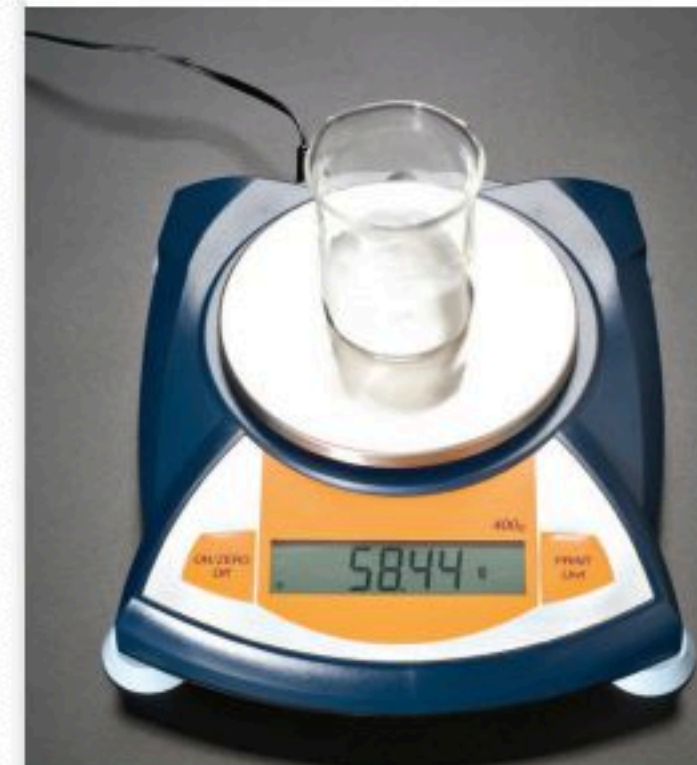
كلوريد الصوديوم ( NaCl )
