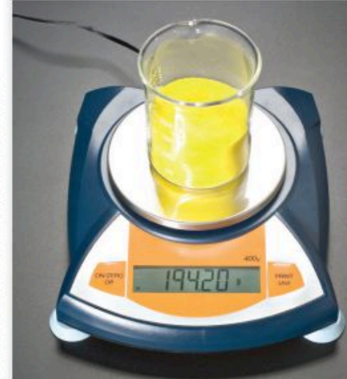
كرومات البوتاسيوم ( K_2CrO_4 )
