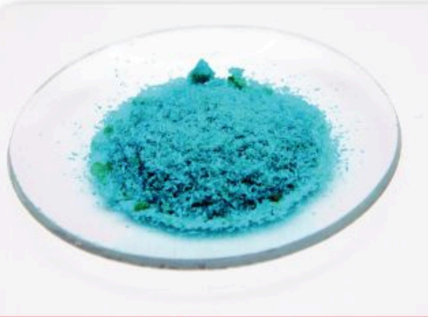
كلوريد النحاس II
