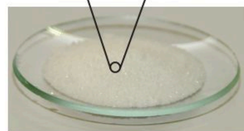
كلوريد الصوديوم NaCl
