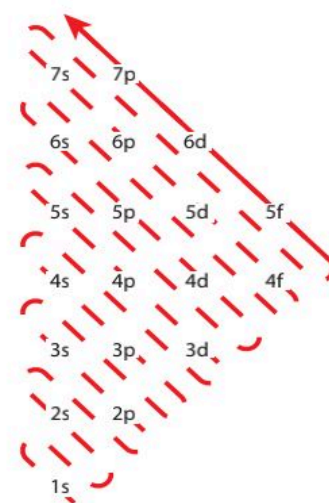
الشكل 4-4 يظهر ترتيب ملء مستويات الطاقة بالإلكترونات.
