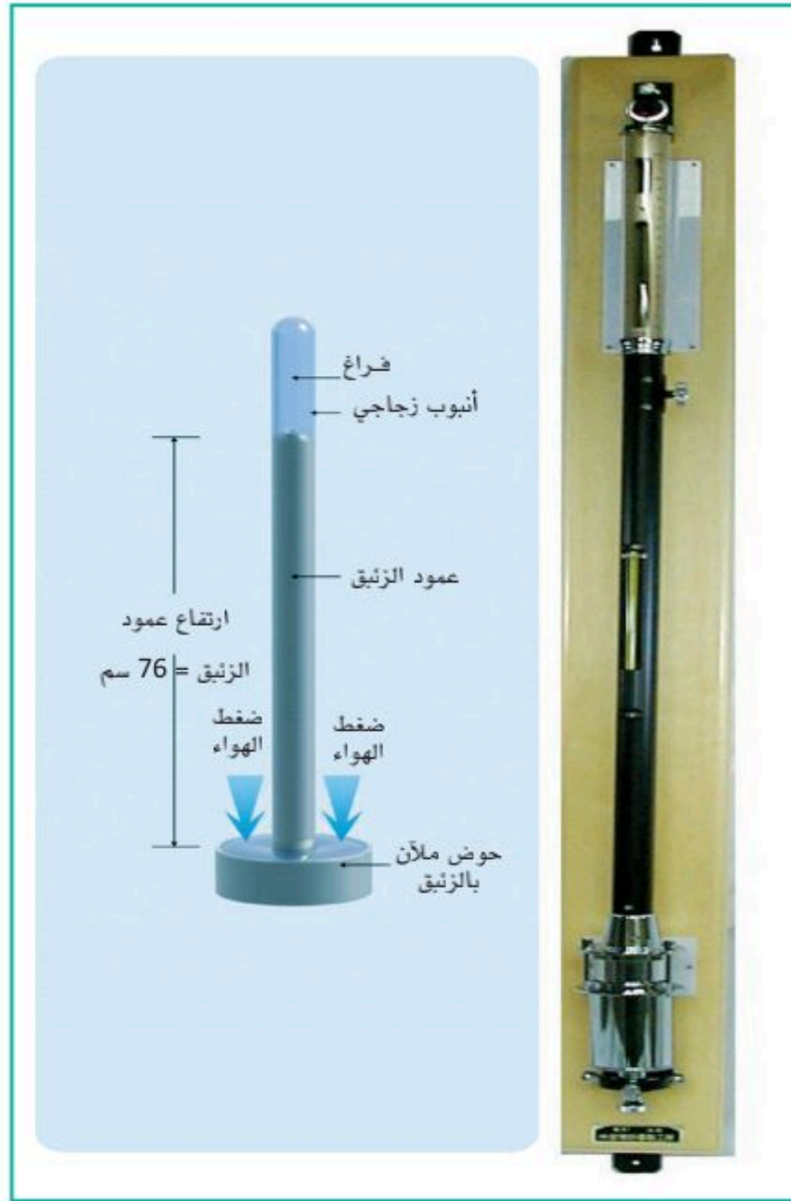
البارومتر الزئبقي
