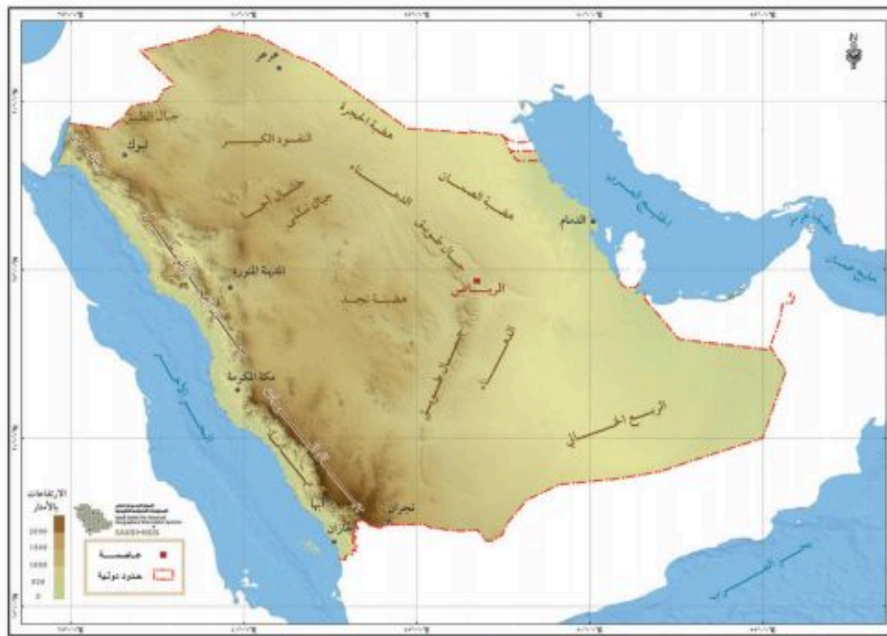
خريطة تضاريسية
