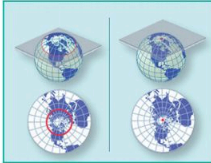
المسقط المستوي
