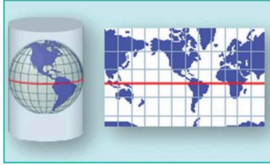
المسقط الأسطواني
