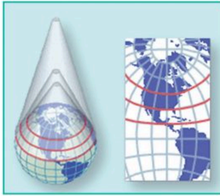
المسقط المخروطي
