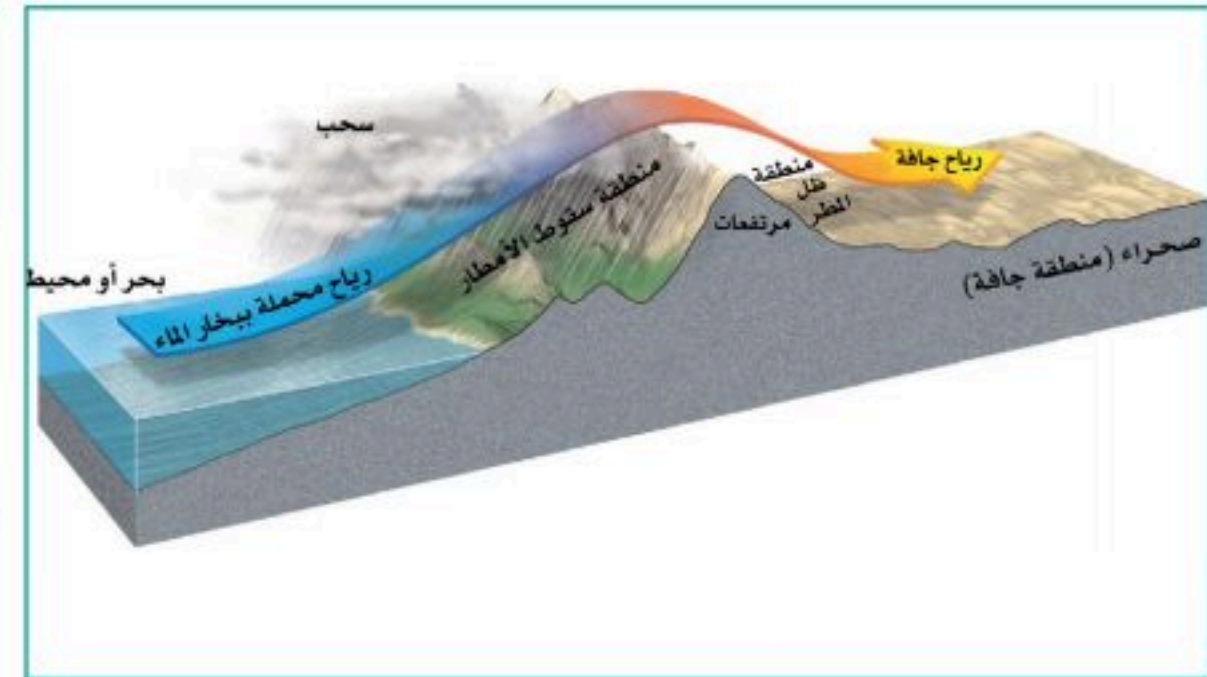
المطر التضاريسي
