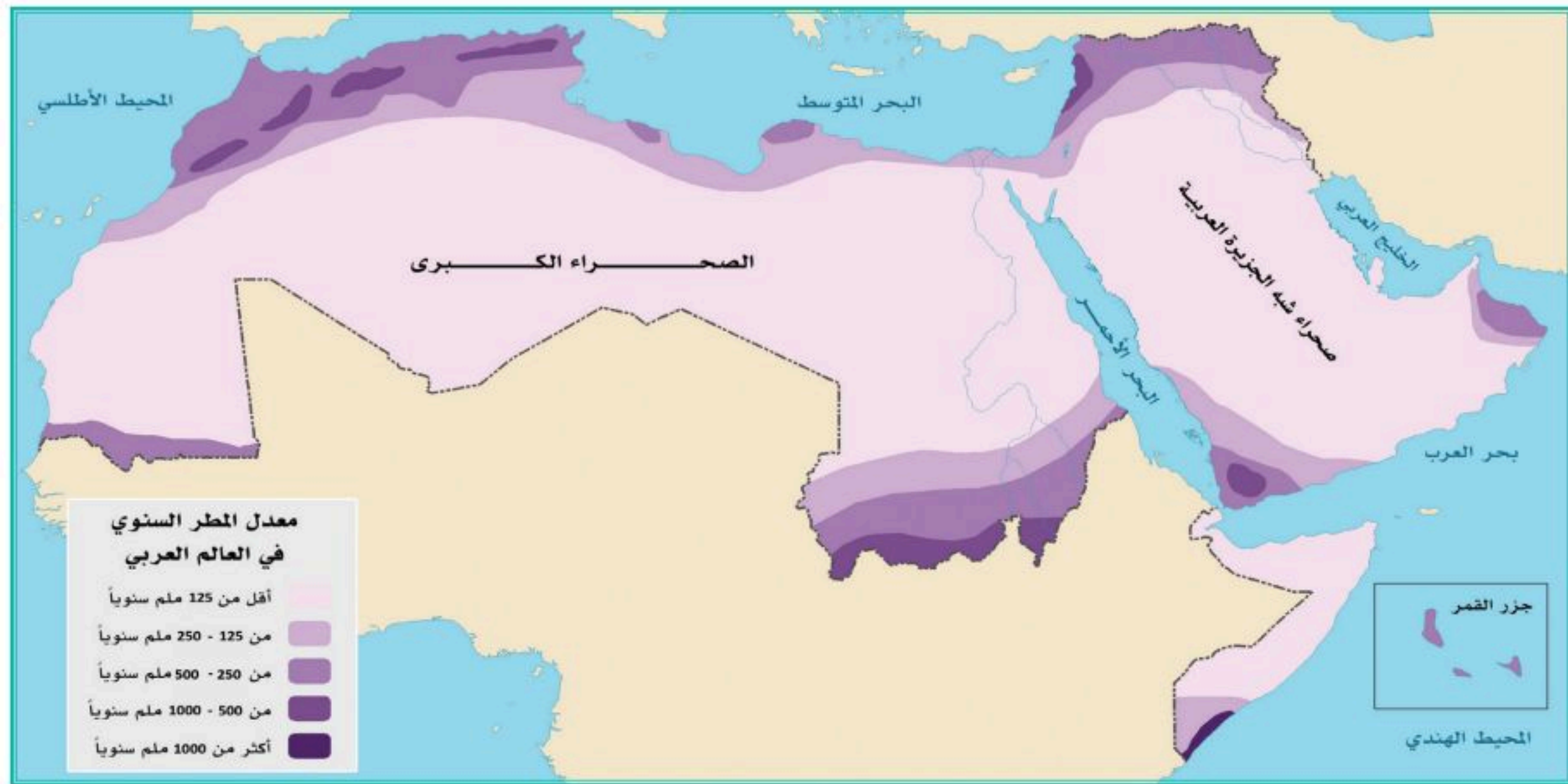
خريطة مناخية
