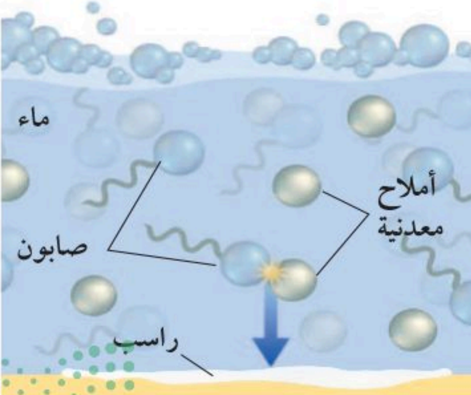
الشكل ٣ تفاعل الأملاح مع الصابون فتشكل راسباً.
