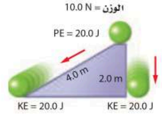
الشكل 10-5 يؤثر المسار الذي يتبعه الجسم حتى يصل الأرض في مقدار الطاقة الحركية النهائية للجسم.
