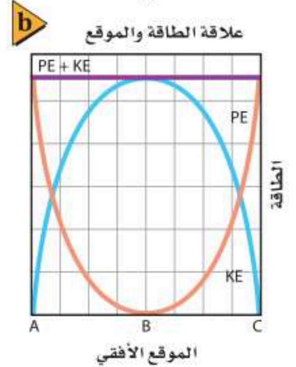
طاقة الوضع. طاقة الحركة. الطاقة الكلية للنظام في أي موقع تساوي مقدار ثابت.
