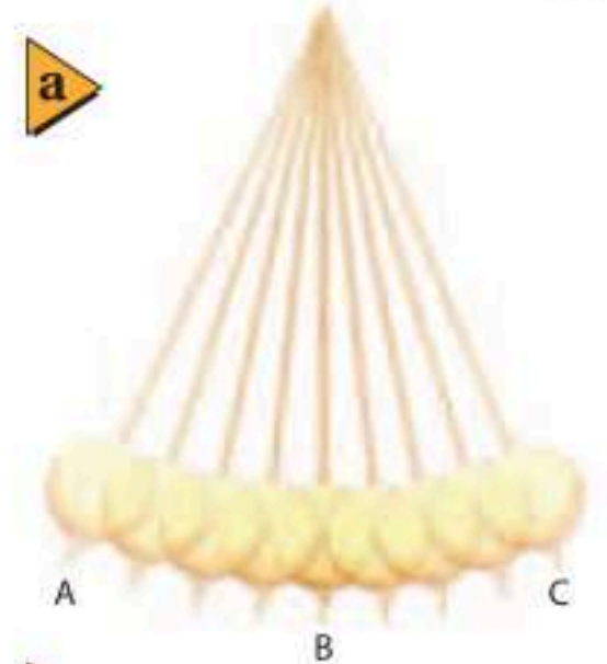
الشكل 11-5 الحركة التوافقية البسيطة لرقاص البندول (a). الطاقة الميكانيكية هي مجموع طاقتي الحركة والوضع وهي مقدار ثابت (b).
