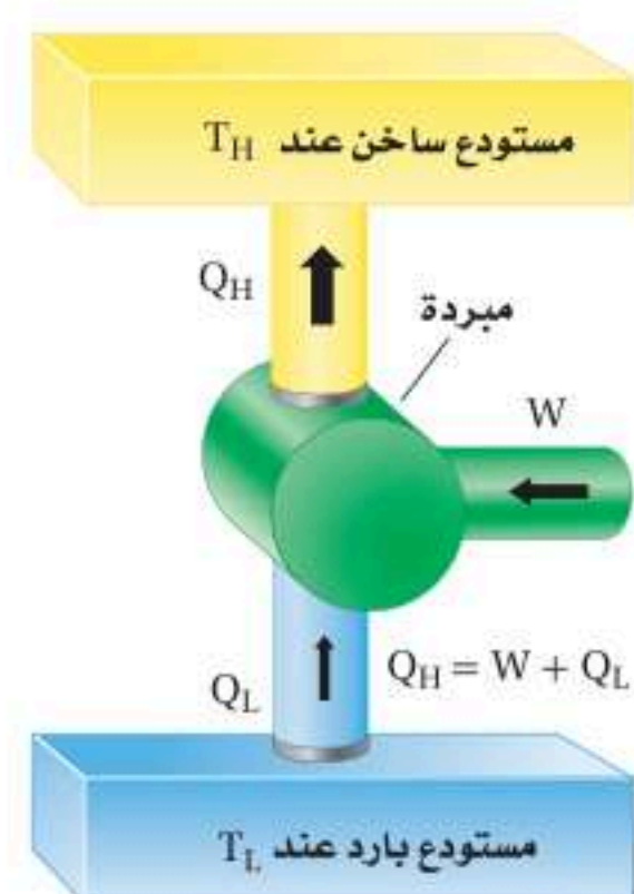
■ الشكل 6-13 يمتص المبرّد الحرارة Q_L من المستودع البارد ويبيّث الحرارة Q_H إلى المستودع الساخن، ببذل شغل W على المبرّد.
