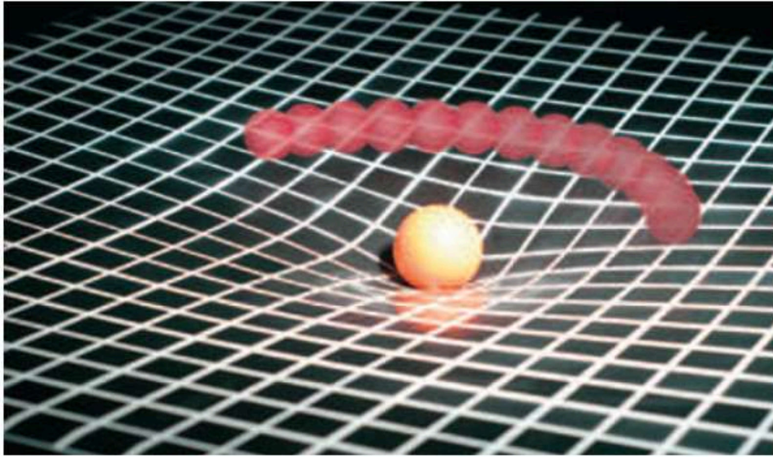
■ الشكل 1-16 تسبب المادة انحناء الفضاء (الزمكان) تماماً كما يؤثر جسم في شبك مطاطي حوله. الأجسام المتحركة بالقرب من الكتلة تسلك مساراً منحنياً في الفضاء. تتحرك الكرة الحمراء في اتجاه حركة عقارب الساعة حول الكتلة المركزية.
