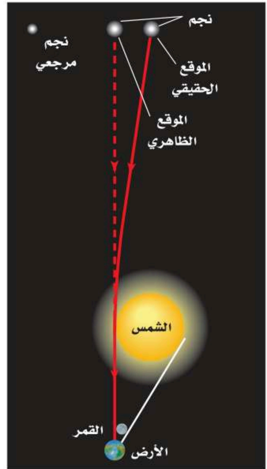
■ الشكل 1-17 الضوء القادم من النجوم البعيدة يتأثر بمجال جاذبية الشمس. الرسم للتوضيح ولا يمثل مقياس رسم حقيقي.
