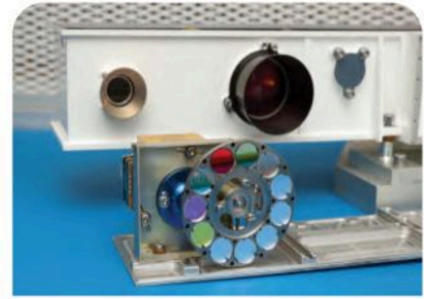
الشكل 11-3 كاميرا مثبتة بأسطوانة فلاتر.
