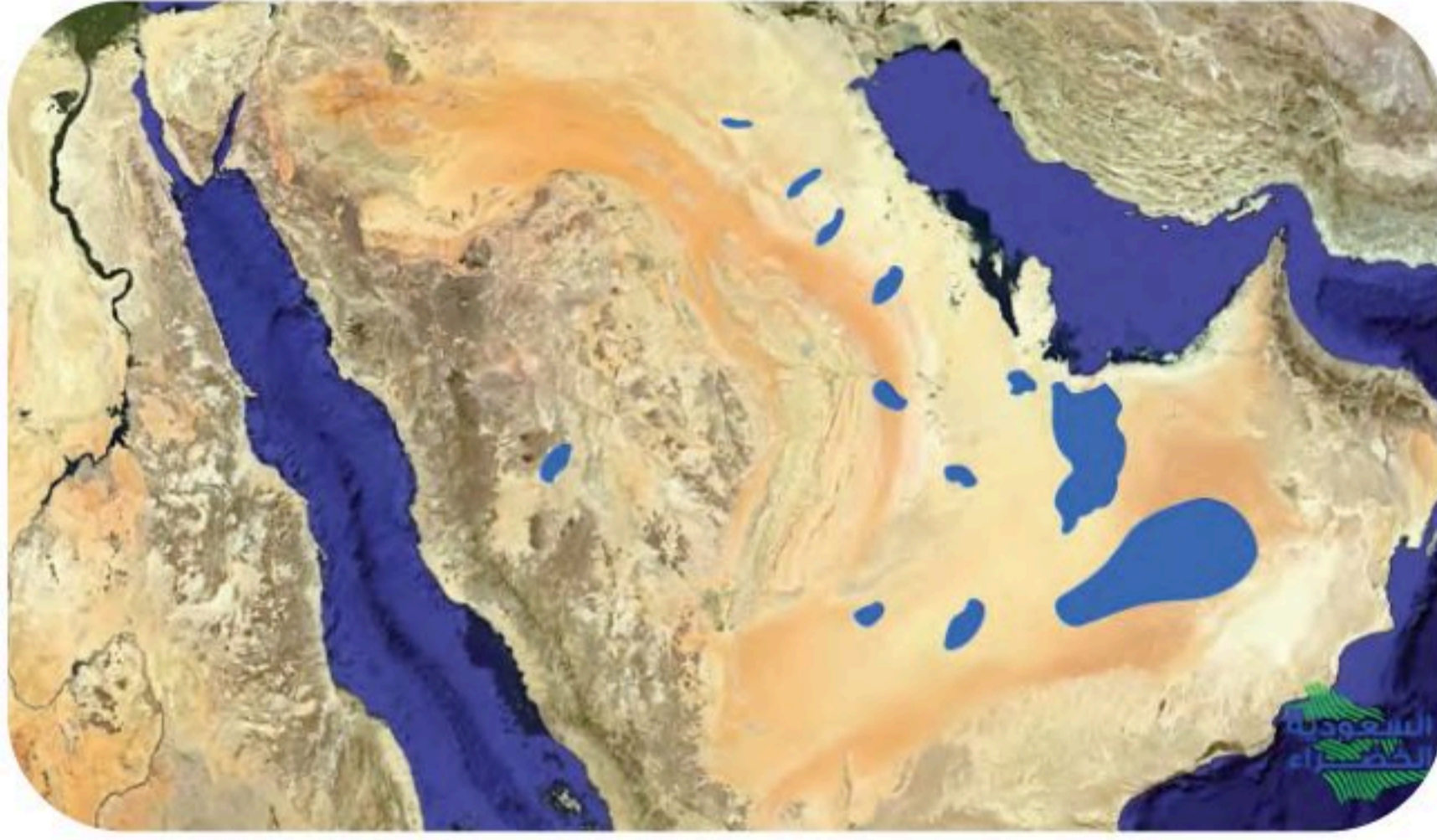
الشكل 10-6 الموقع الجغرافي لبعض السبخات في المملكة العربية السعودية.
