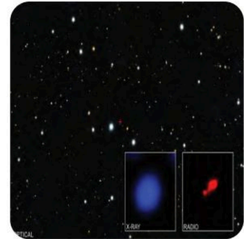
الشكل 16-3 كوازارات. المصدر: وكالة ناسا.
