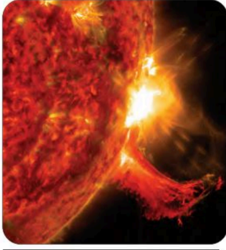
الشكل 9-2 التوهجات الشمسية.
