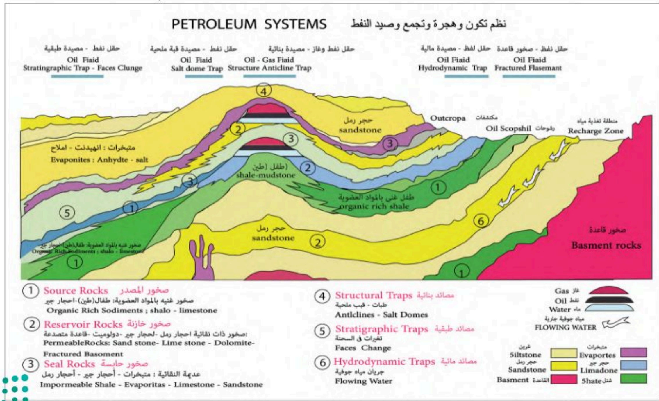
الشكل 1-5 النظام النفطي.
