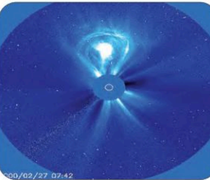
الشكل 11-2 الانبعاث الكتلي الإكليلي.
