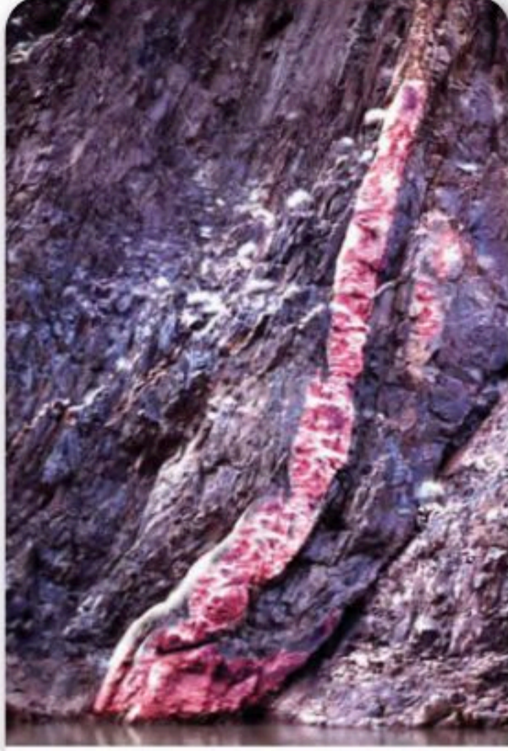
الشكل 4-20 بحسب مبدأ القاطع والمقاطع فإن القواطع النارية أحدث من صخور الشيست.
