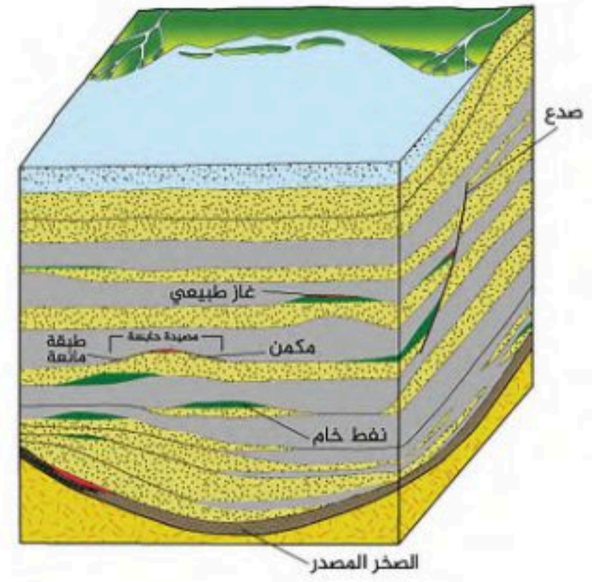
الشكل 2-5 صخر المصدر.
