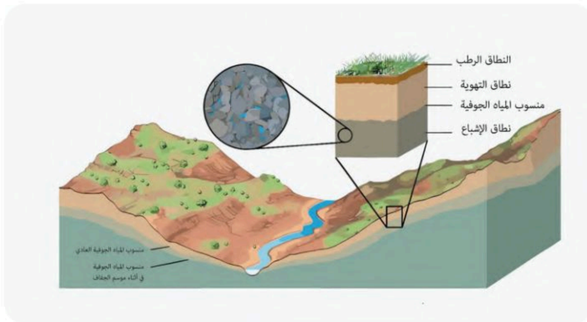
الشكل 14-6 المياه الجوفية.
