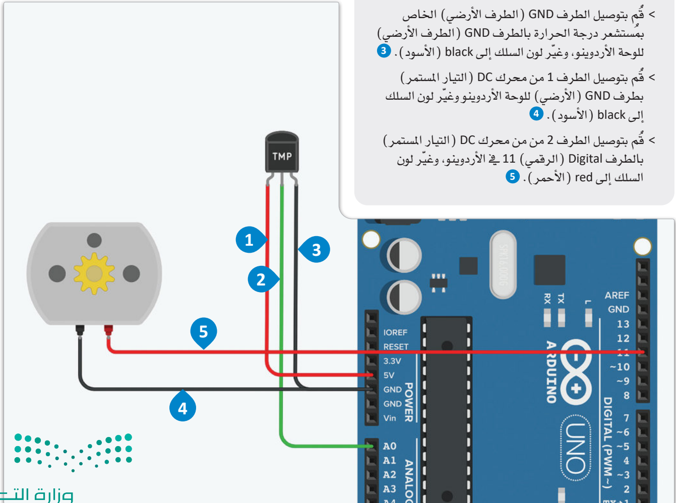
شكل 6.16: توصيل الدائرة
