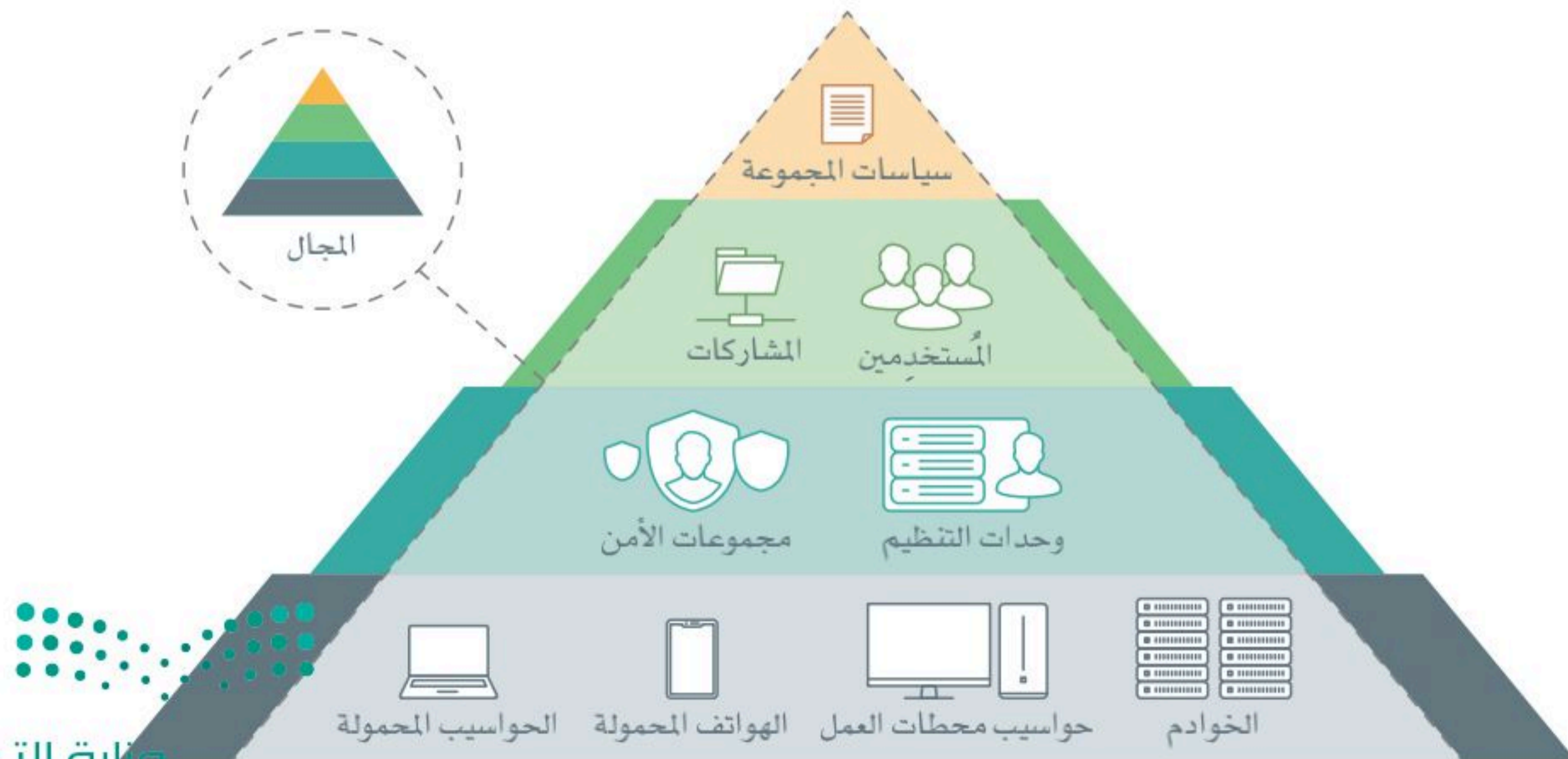
شكل 1.17: هيكلية الدليل النشط
