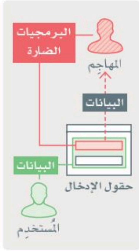
شكل 1.9: مثال على هجوم البرمجة العابرة للمواقع (XSS)
