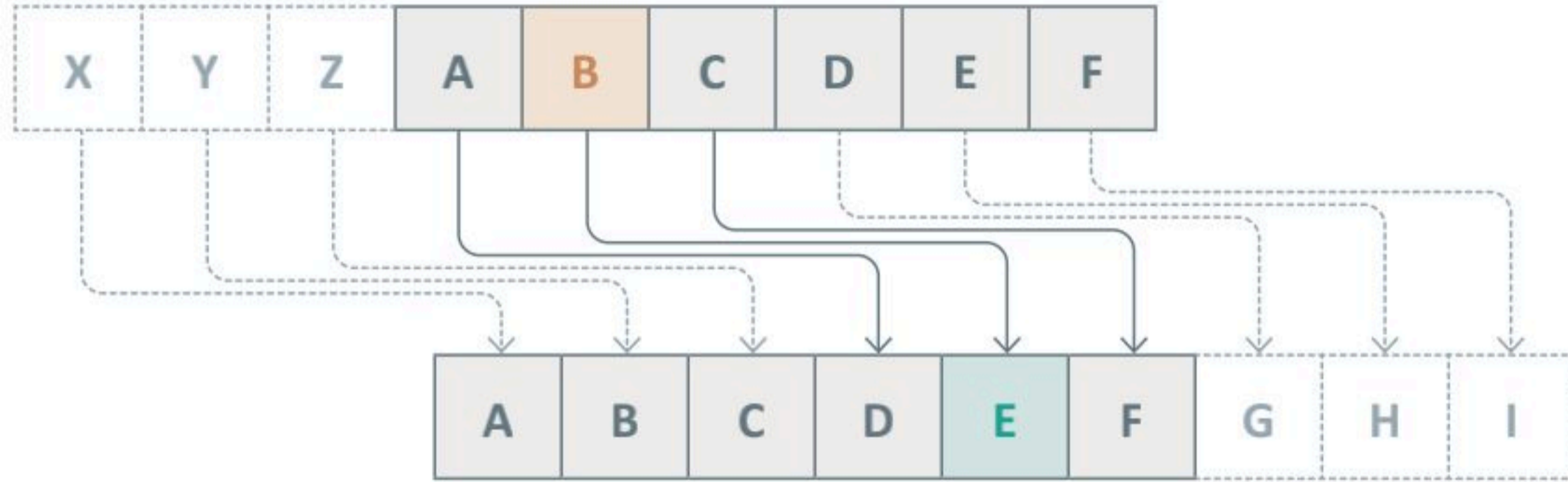
شكل 3.7: تمثيل خوارزمية تشفير قيصر باستخدام مفتاح = 3
