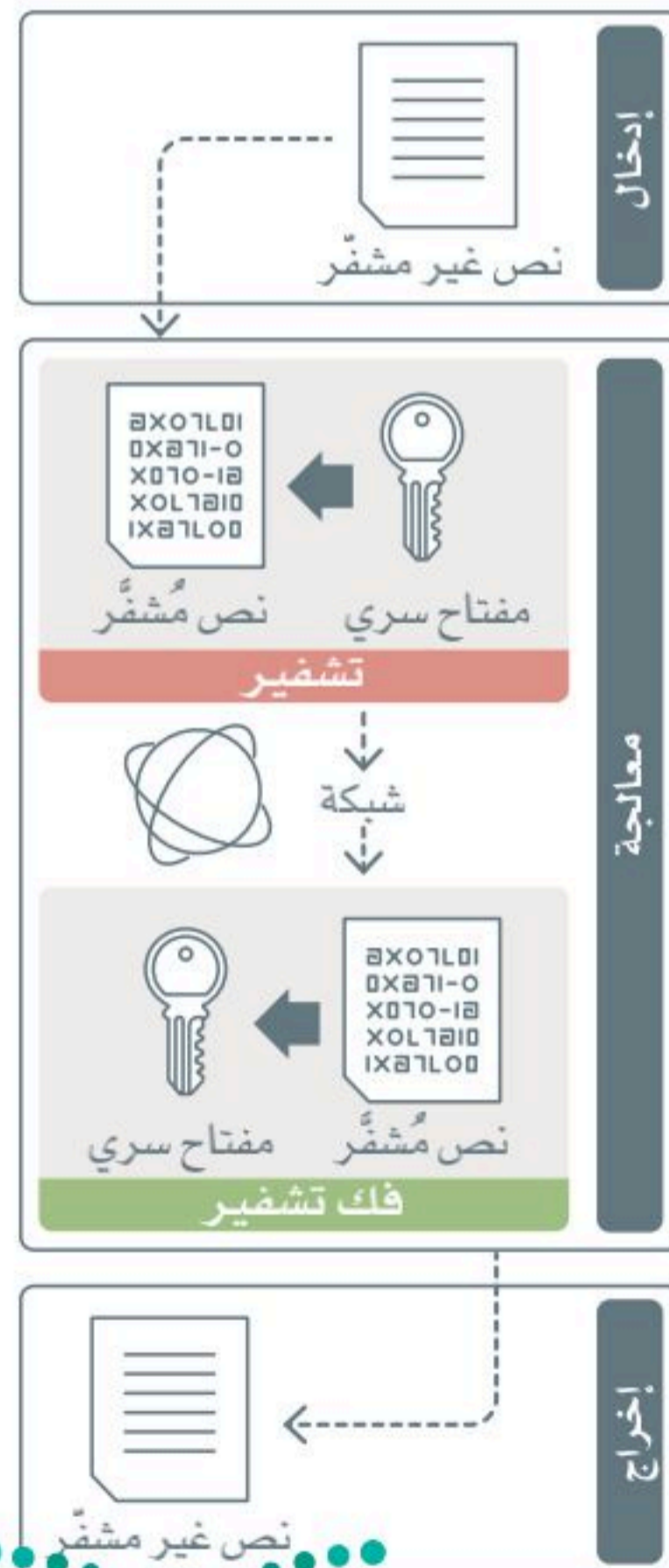
شكل 3.3: مثال عملي لتشفير وفك تشفير قياسية
