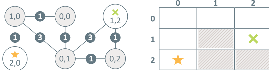
شكل 2.21: المتاهة ومخططاتها الموزون
