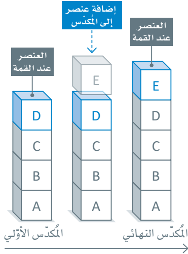
شكل 1.13: عملية إضافة عنصر إلى المُكدّس
