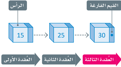
شكل 1.30: الوصول إلى العُقدة الثالثة في القائمة المترابطة
