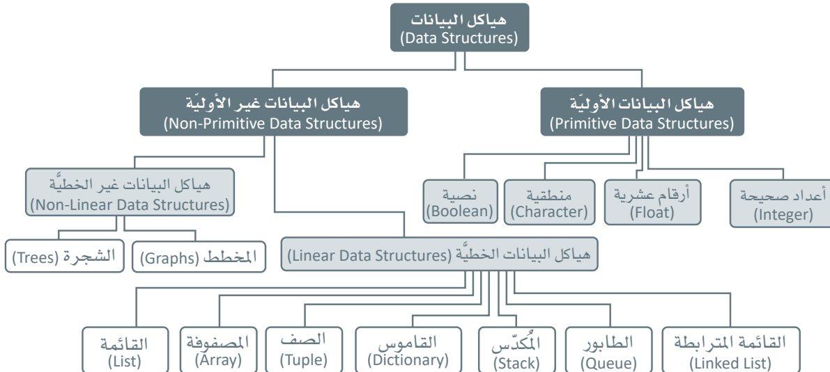
شكل 1.11: مخطط هياكل البيانات
