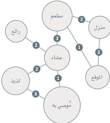
شكل 3.27: مثال على مُخطَّط موزون لـ Networkx
