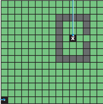
شكل 2.23: خلية البداية والخلية المستهدفة للمتاهة
