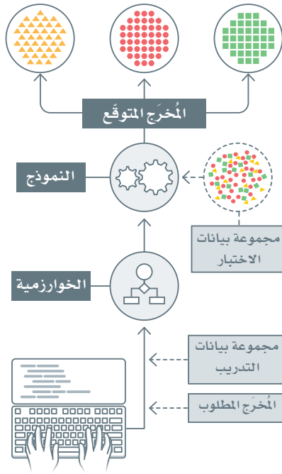
شكل 3.2: تمثيل التعلُّم الموجَّه
