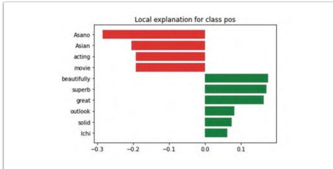
شكل 3.11: الكلمات التي أثرت على القرار الخاطئ
