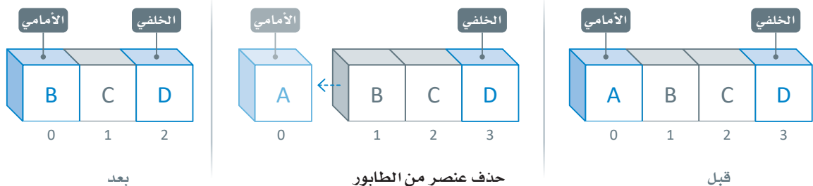
شكل 1.24: عملية حذف عنصر من الطابور
