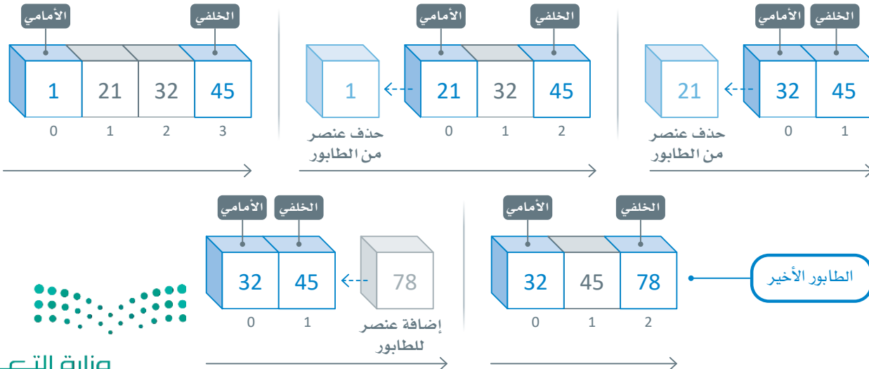
شكل 1.25: مثال توضيحي لمفهوم الطابور
