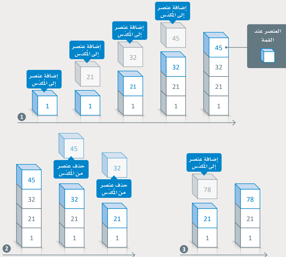
شكل 1.15: مثال على المكدّس
