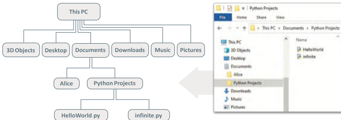
شكل 1.37: تنظيم الملفات في نظام التشغيل
