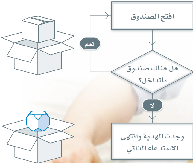
شكل 2.1: مثال على الاستدعاء الذاتي
