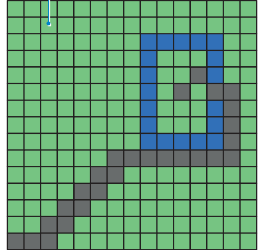
شكل 2.24: مقارنة بين حلّي خوارزميتي البحث بأولوية الاتساع والبحث بأولوية الأفضل
