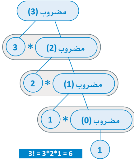
شكل 2.4: شجرة الاستدعاء الذاتي
