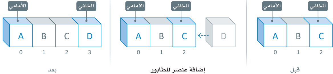
شكل 1.23: عملية إضافة عنصر للطابور
