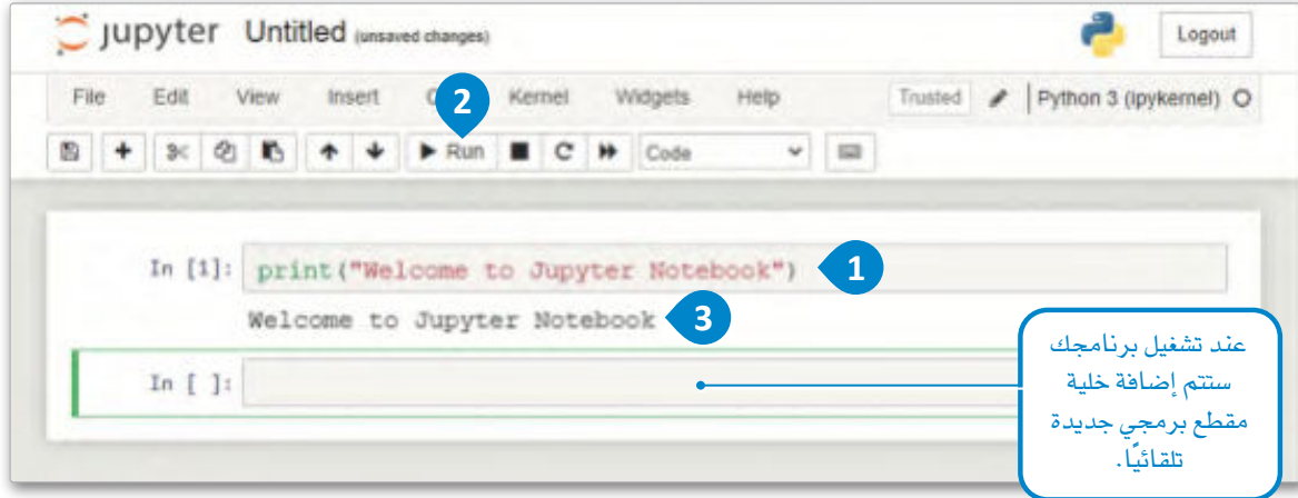
شكل 1.18: إنشاء برنامج في مفكرة جوبيتر
