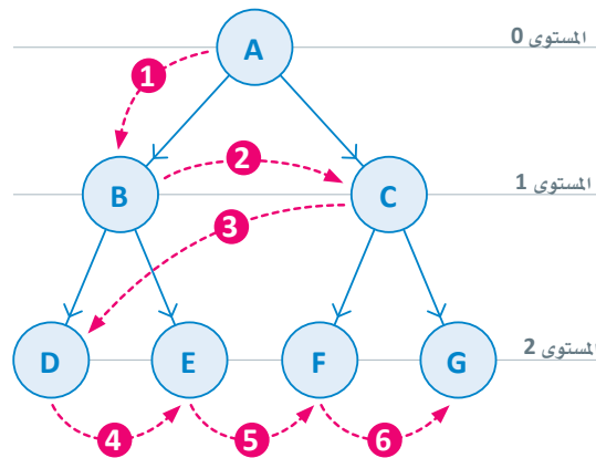
شكل 2.6: خوارزمية البحث بأولوية الاتساع (BFS)
