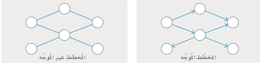
شكل 1.43: المخطَّط المُوَّجَّه و المخطَّط غير المُوَّجَّه
