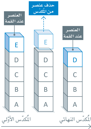
شكل 1.14: عملية حذف عنصر من المُكدّس
