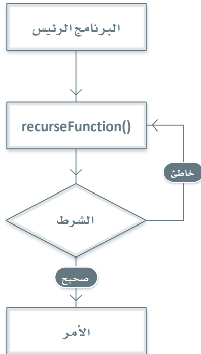
شكل 2.2: تمثيل الاستدعاء التكراري
