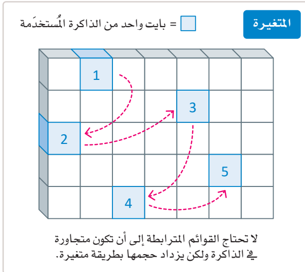
شكل 1.26: مثال على تخصيص الذاكرة الثابتة والمتغيرة.
