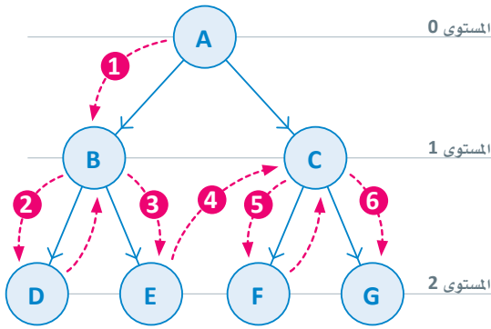
شكل 2.7: خوارزمية البحث بأولوية العمق (DFS)
