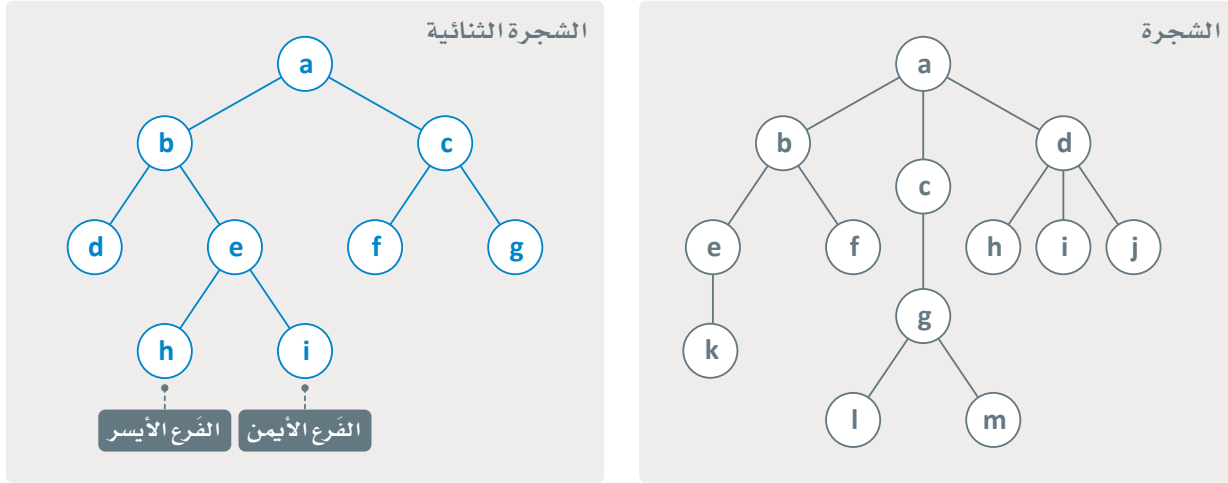
شكل 1.40: الشجرة والشجرة الثنائية
