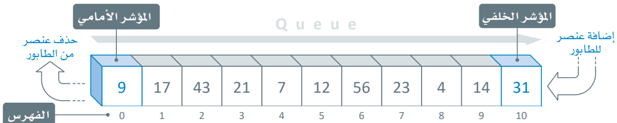
شكل 1.22: العمليات في الطابور
