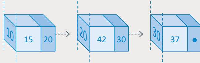
شكل 1.31: المؤشرات في القائمة المترابطة
