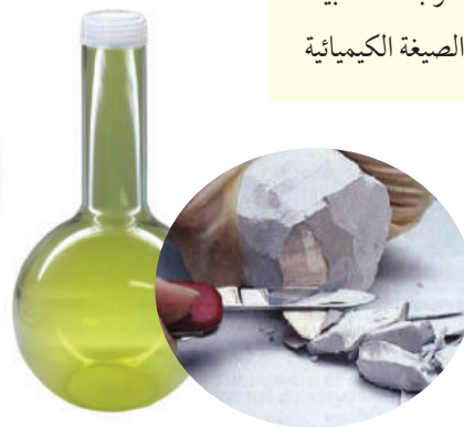
غاز كلور
