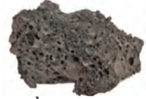
الْجِرَانِيْتُ
