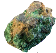
الْفُلُورَايْتُ
