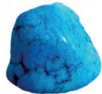
الْتَرْكُوَازُ
